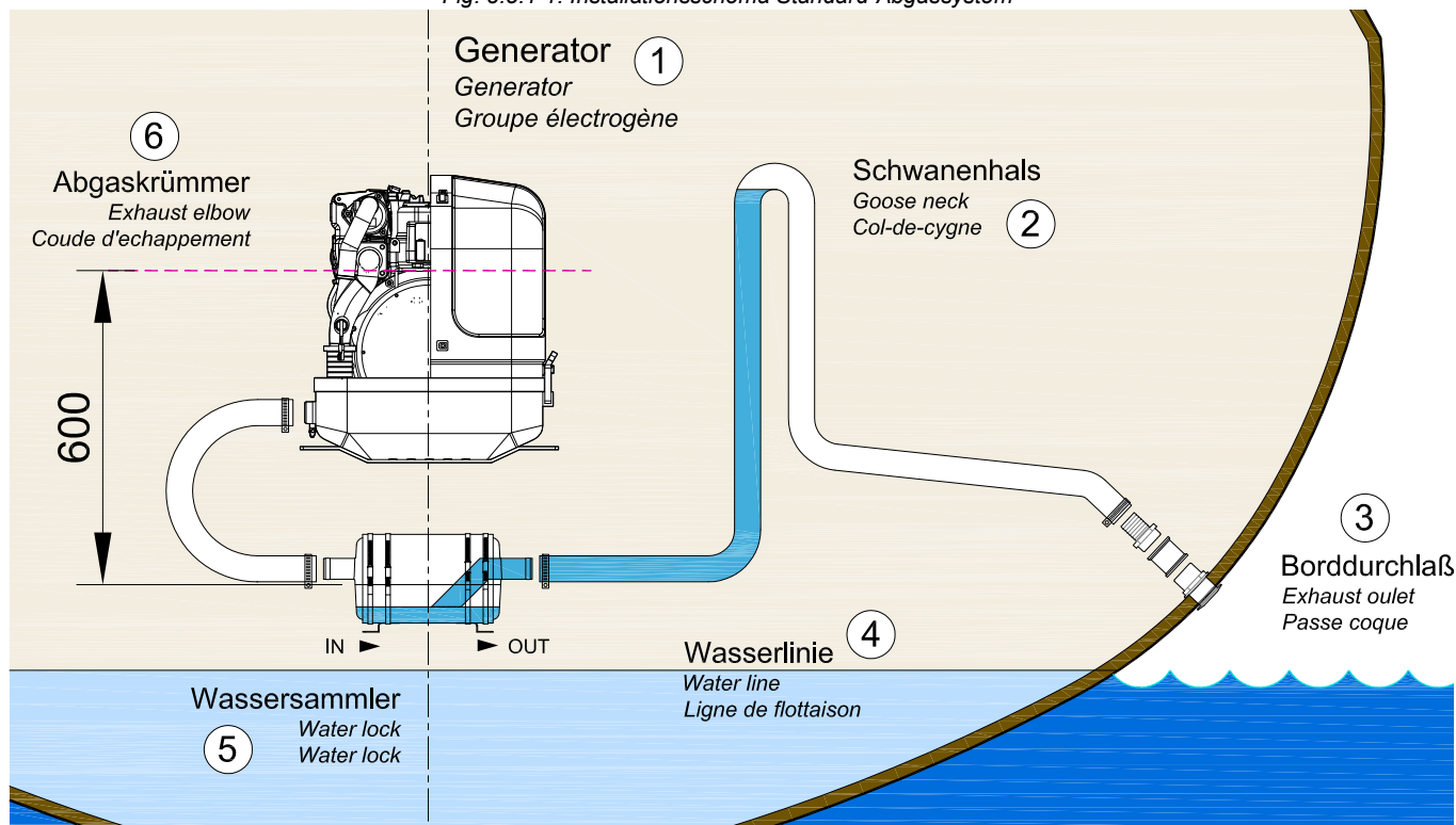
Fig. 8.5.1-1: Installationsschema Standard-Abgassystem
