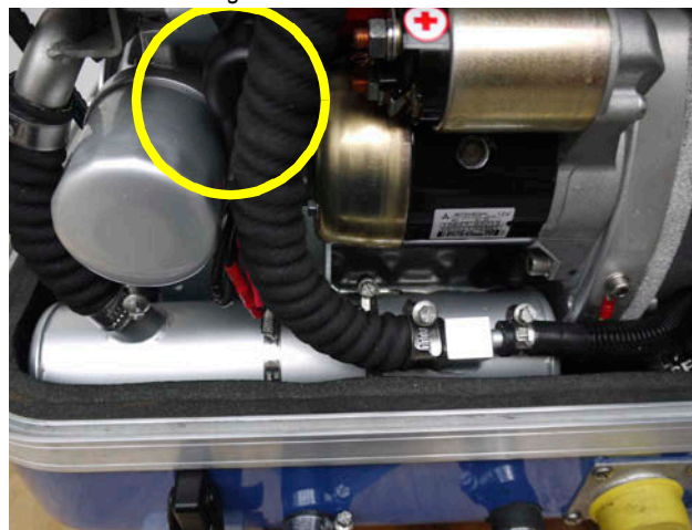
Fig. 7.3.6-4: Öldruckschalter
