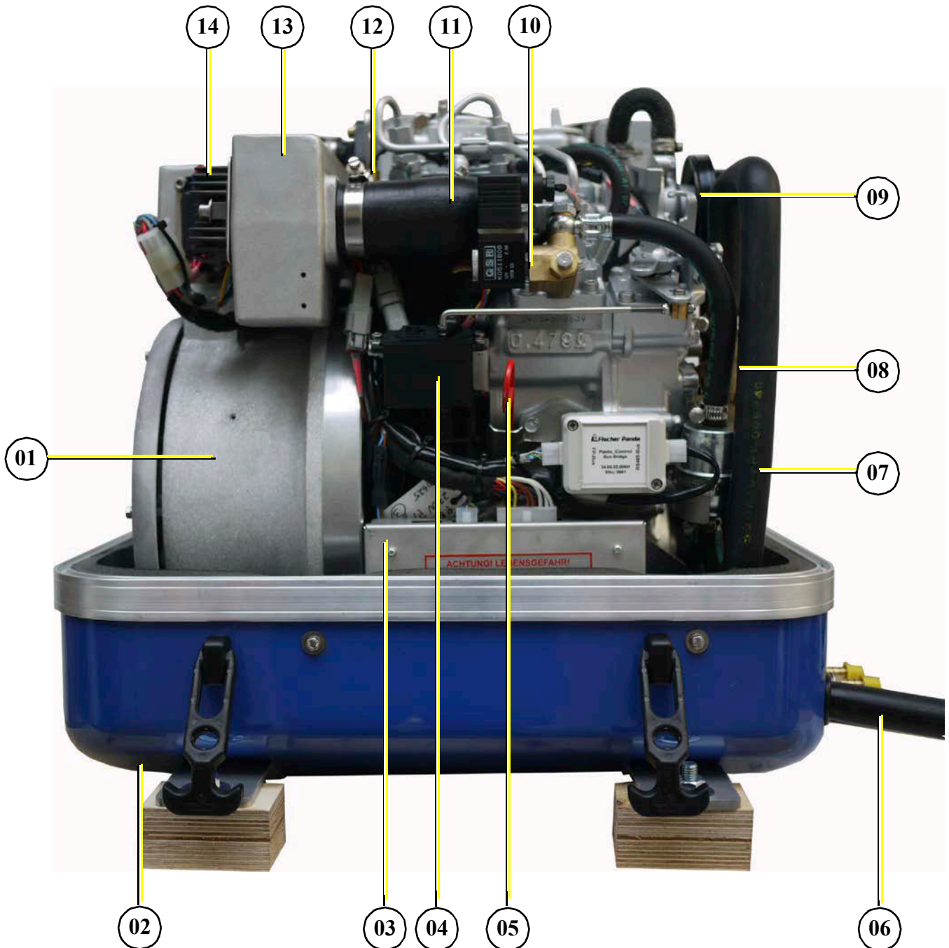
Fig. 7.2.2-1: Seitenansicht Links
