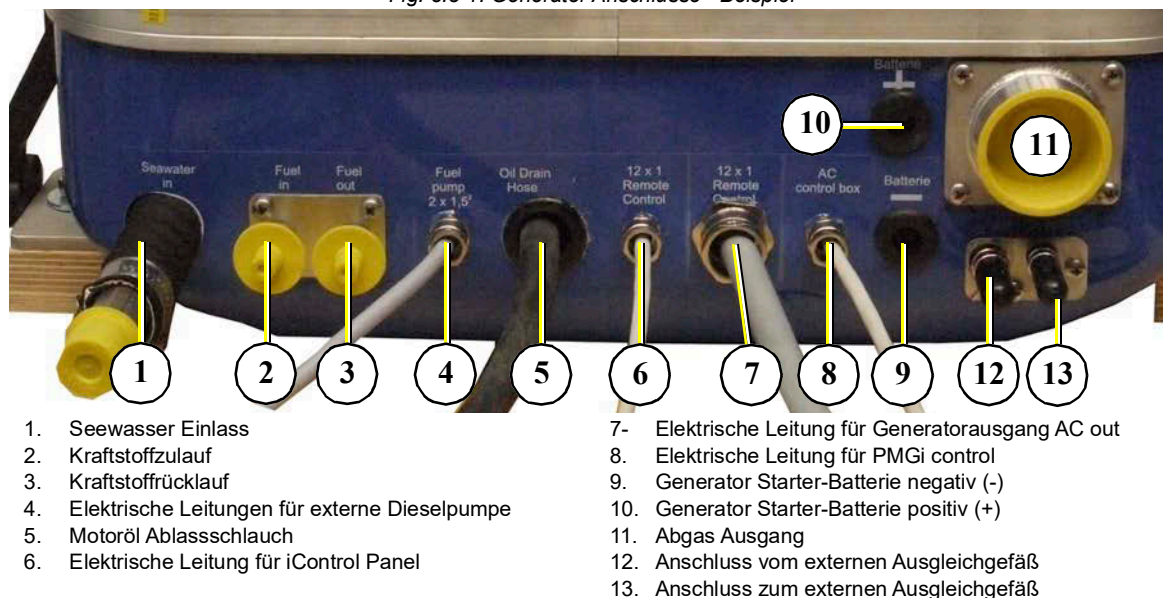
Fig. 8.3-2: Generator Anschlüsse - Beispiel
