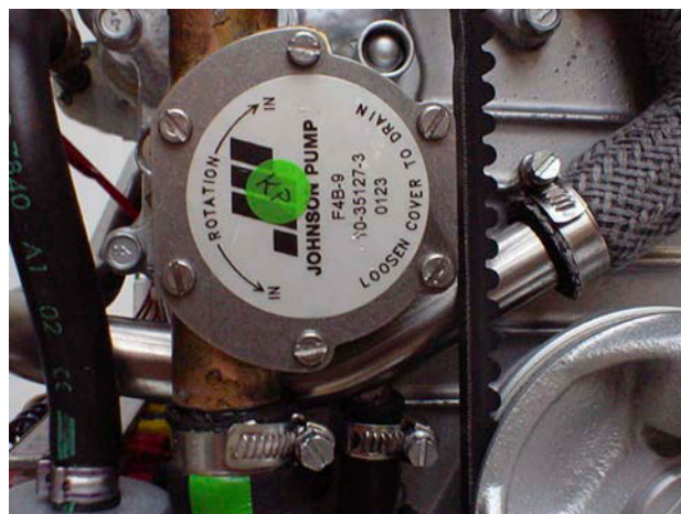
Fig. 10.4.3-3: Gehäuse Seewasserpumpe
