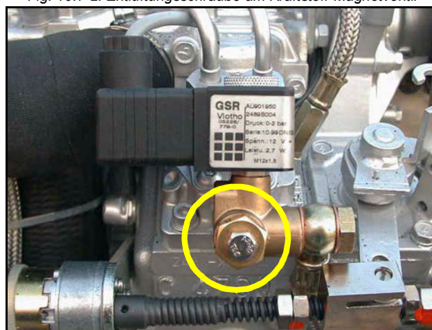
Fig. 10.7-2: Entlüftungsschraube am Kraftstoff-Magnetventil
