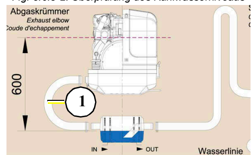
Fig. 8.6.3-2: Überprüfung des Kühlwasserniveaus
