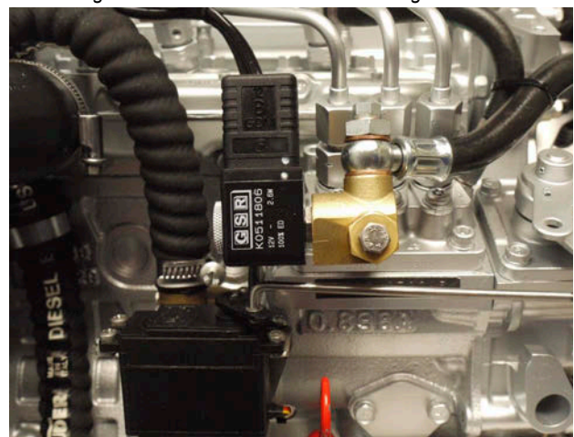
Fig. 11.4.1-1: Elektrisches Kraftstoffmagnetventil
