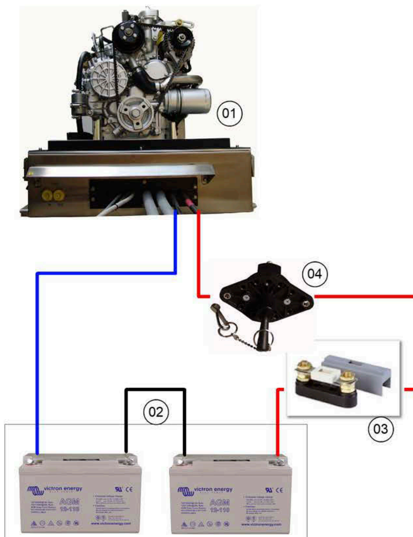
Fig. 8.10.3-2: Starterbatterieanschluss 24 V - Schema
