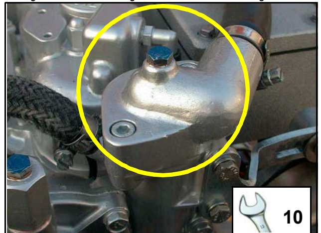
Fig. 10.5.3-3: Entlüftungsschraube am Thermostatgehäuse
