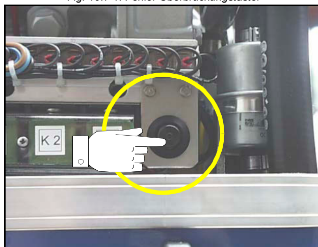
Fig. 10.7-1: Fehler-Überbrückungstaster
