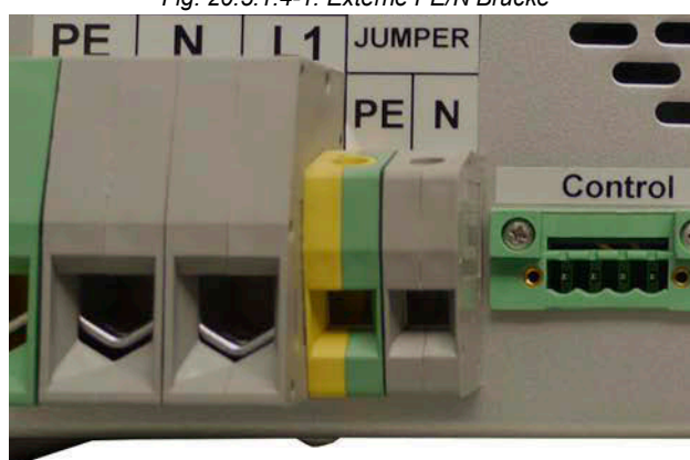
Fig. 20.5.1.4-1: Externe PE/N Brücke
