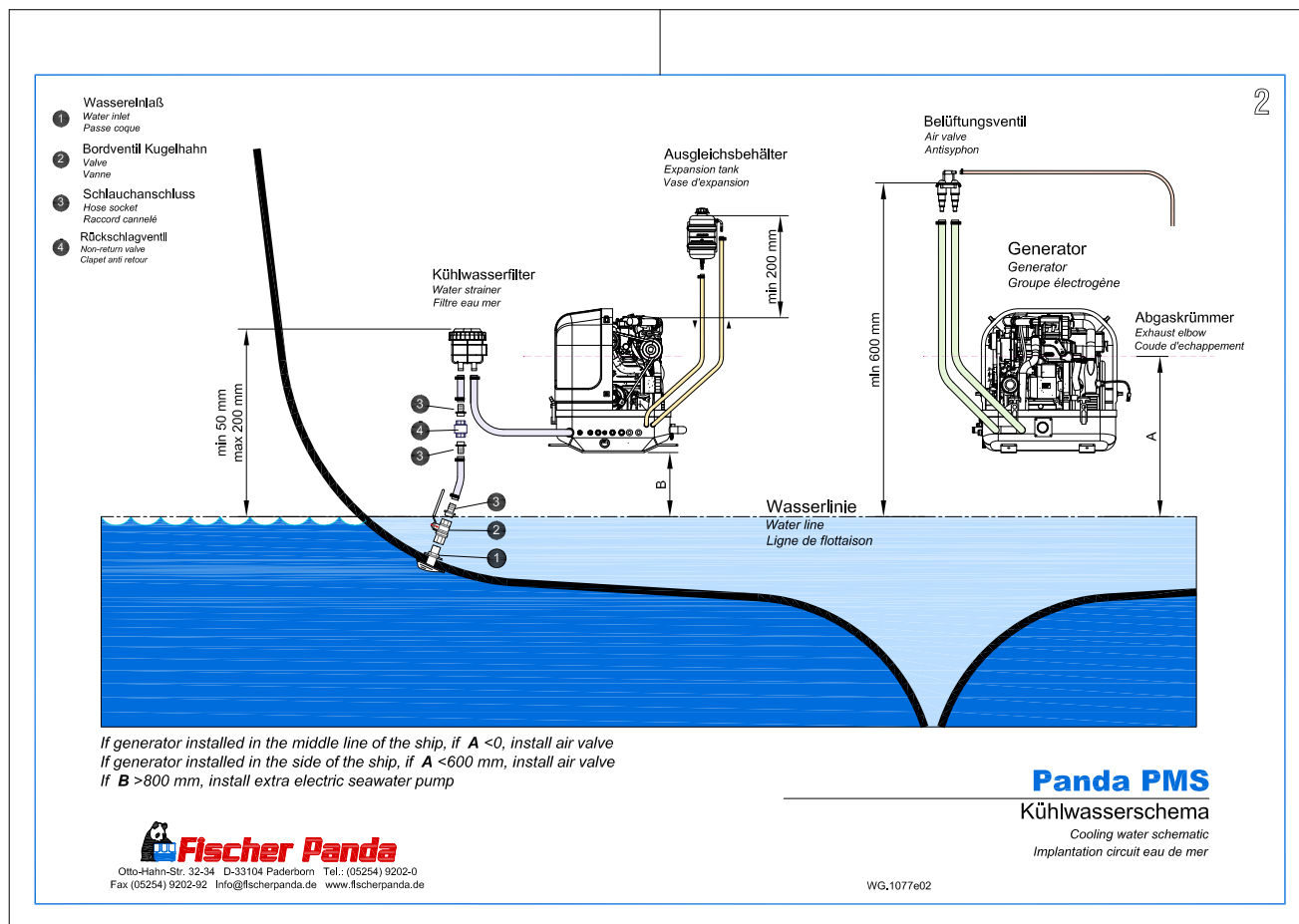
Fig. 8.4.4.1-1: Seewasser Installationschema
