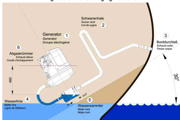
Fig. 8.6.3.1-3: Schräglage 30 Grad
