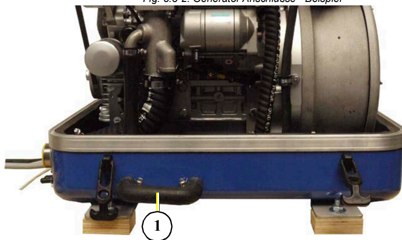
Fig. 8.3-2: Generator Anschlüsse - Beispiel
