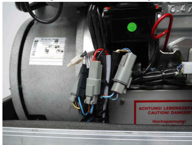
Fig. 7.3.6-3: Thermosensor Wicklung
