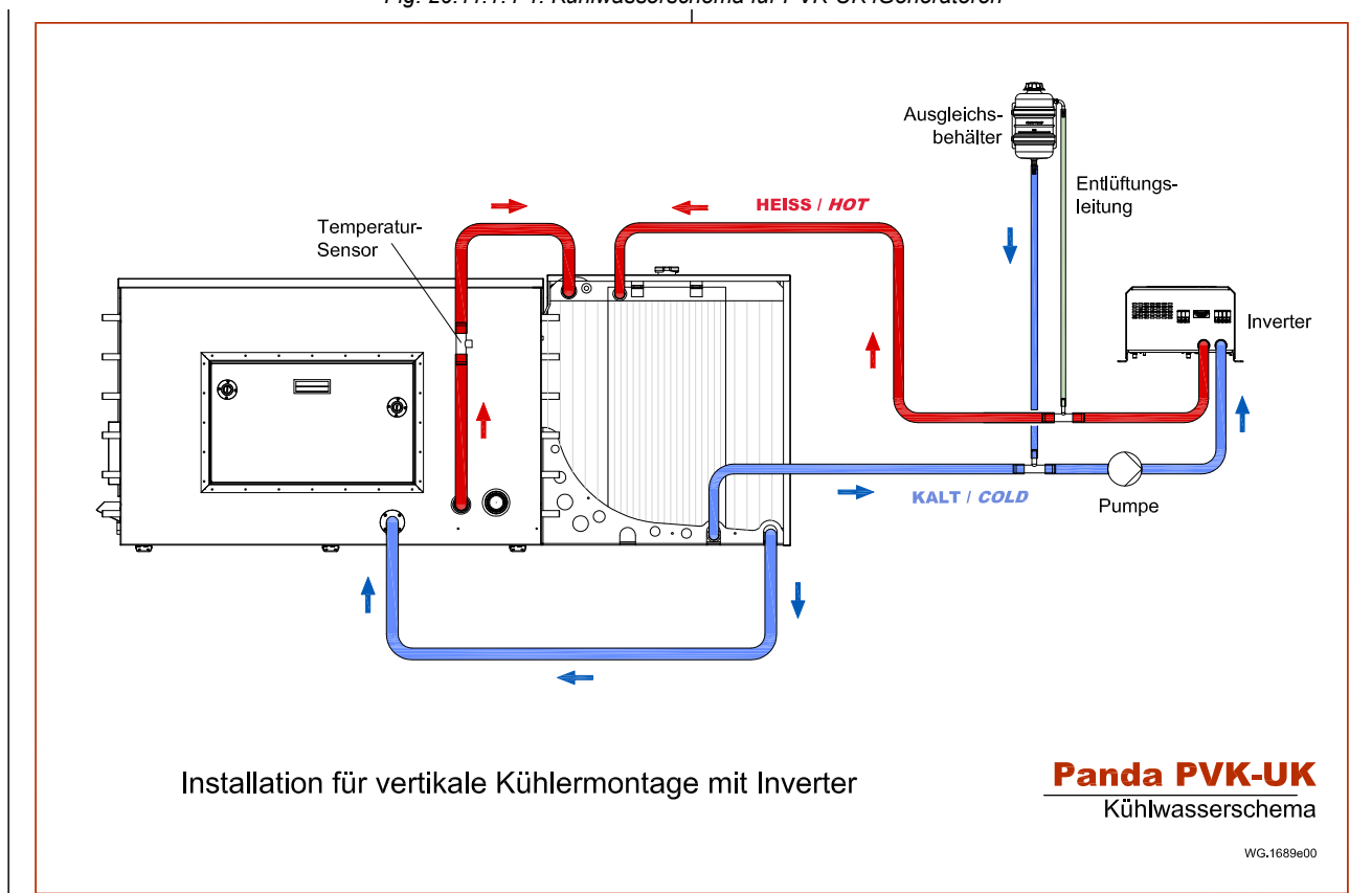
Fig. 20.11.1.4-1: Kühlwasserschema für PVK-UK iGeneratoren
