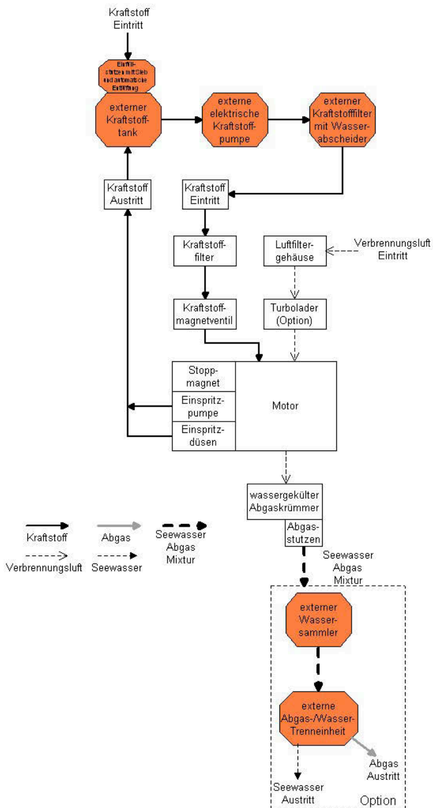
Fig. 7.3.3-1: Kraftstoff-, Verbrennungsluft- und Abgassystem
