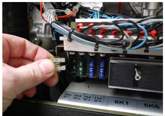
Fig. 10.12-3: Sicherung
