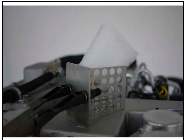
Fig. 10.7.1-4: Luftfiltergehäuse mit Schnellwechselhalter
