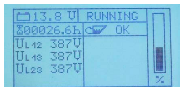
Fig. 15.3.3.4-4: Inverterseite Außenleiterspannungen
