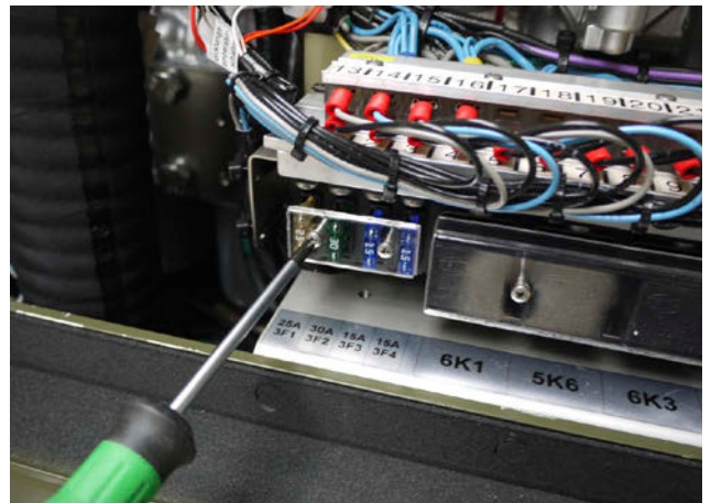
Fig. 10.12-1: Sicherung
