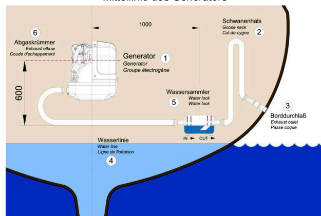
Fig. 8.6.3.2-3: Abgaswassersammler 1000 mm neben der Mittellinie des Generators
