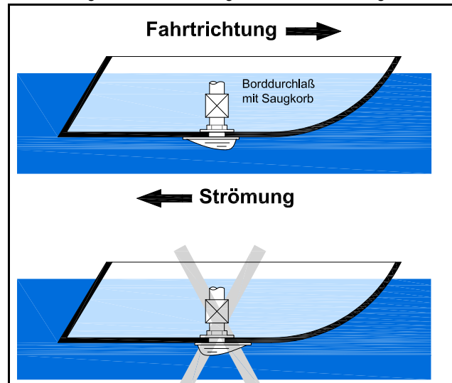
Fig. 8.4.2-1: Anordnung der Borddurchführung
