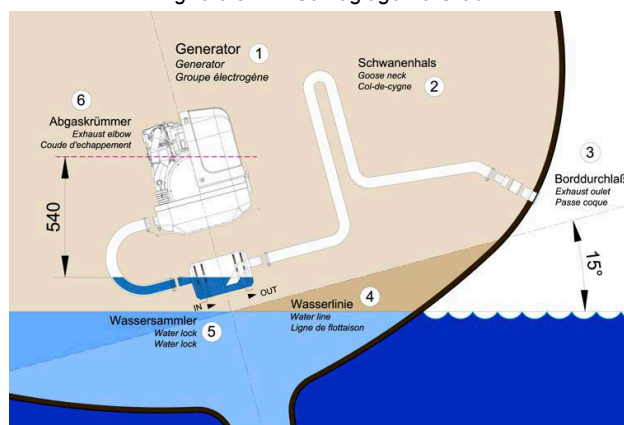
Fig. 8.6.3.1-2: Schräglage 15 Grad
