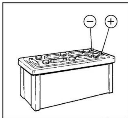
Fig. 10.10.1.1-1: Batterie
