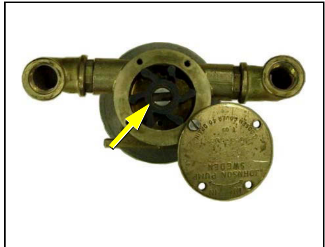
Fig. 10.4.3-4: Impeller
