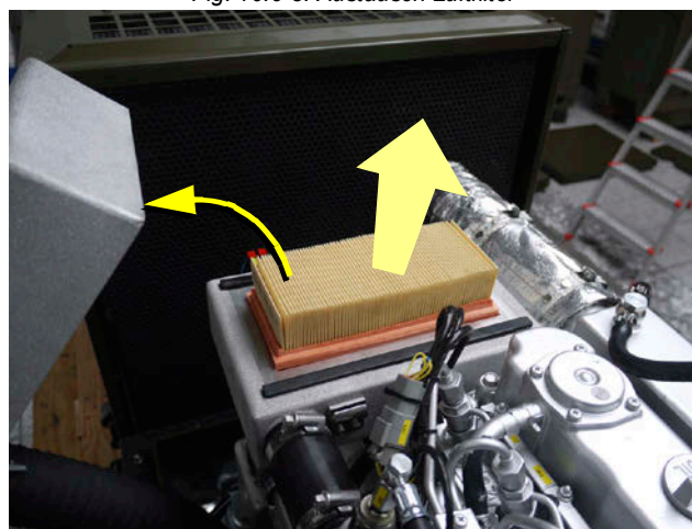
Fig. 10.6-3: Austausch Luftfilter
