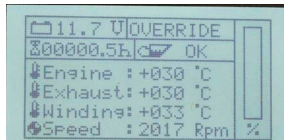
Fig. 15.3.3.3-1: Standard-Displayseite während des Override-Modus
