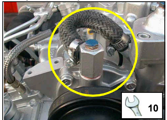
Fig. 10.5.3-2: Entlüftungsschraube am Rohrstutzen
