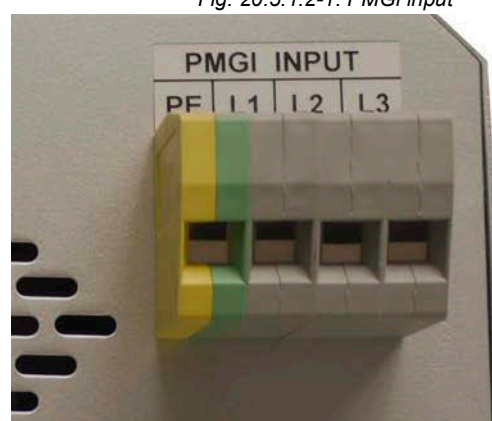
Fig. 20.5.1.2-1: PMGi input
