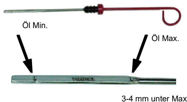
Fig. 10.8.1-1: Ölpeilstab - Beispiel
