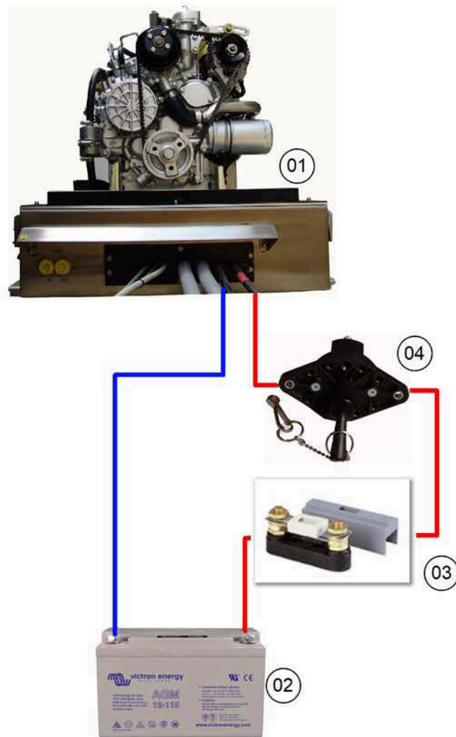
Fig. 8.10.3-1: Starterbatterieanschluss 12 V- Schema
