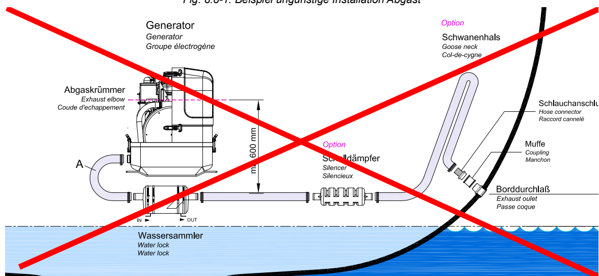
Fig. 8.8-1: Beispiel ungünstige Installation Abgas
