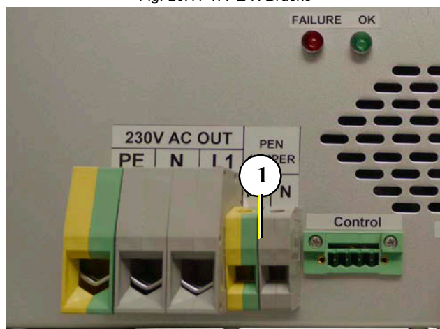
Fig. 20.11-1: PE-N Brücke
