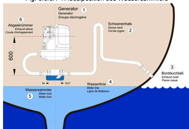
Fig. 8.6.3.1-1: Idealposition des Wassersammlers
