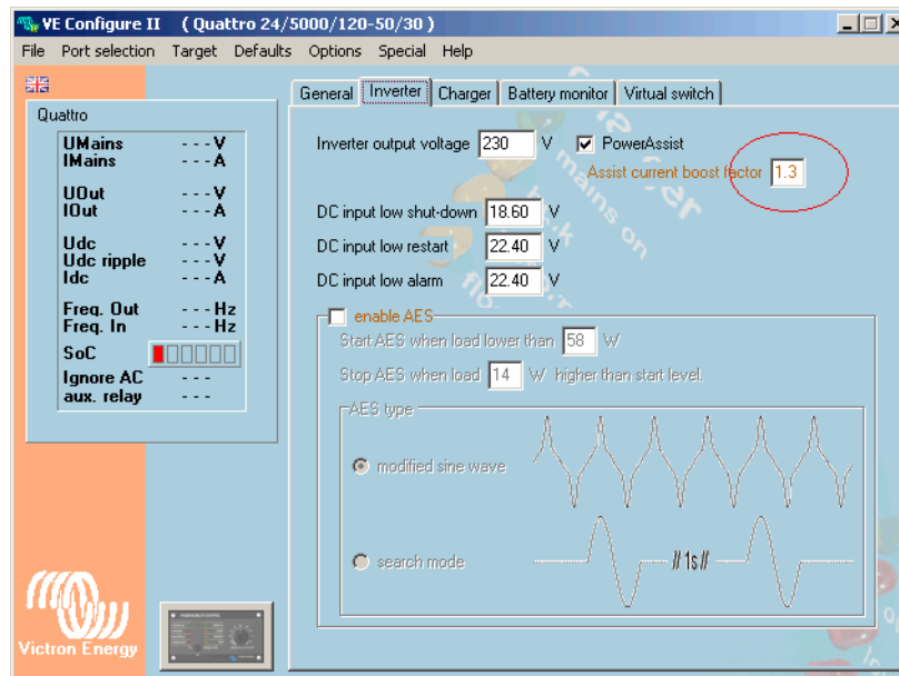
Fig. 20.7.2-1: Einstellungen in der Victron VE Configure II Software
