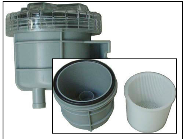
Fig. 10.4.1-1: Seewasserfilter
