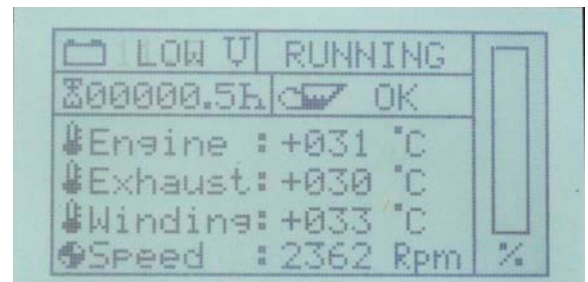
Fig. 18.1.1-1: Warnung „Batteriespannung zu niedrig“
