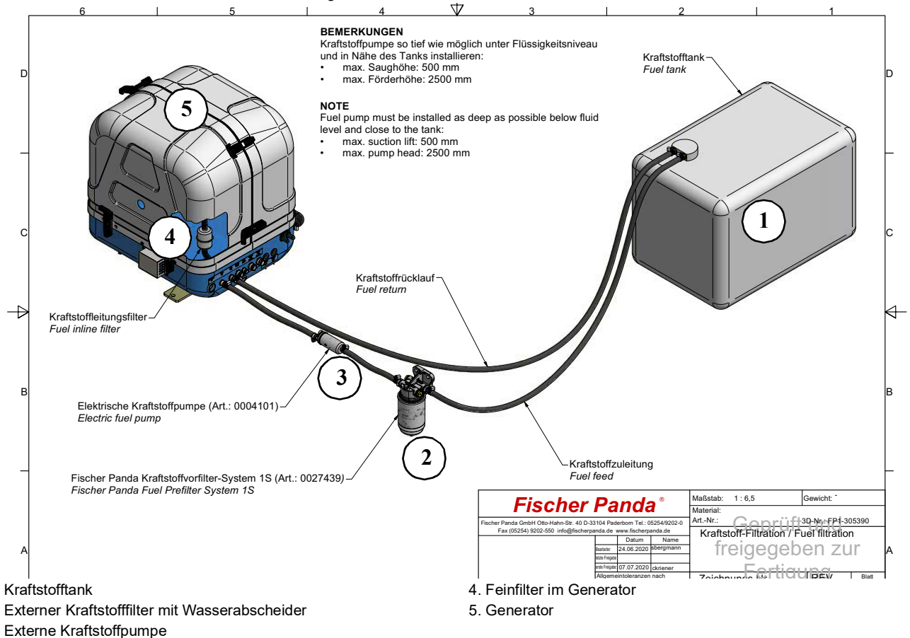
Fig. 8.9.1-2: Kraftstoffanschluss - Schema
