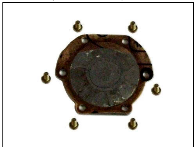
Fig. 10.4.3-6: Deckel Pumpenwelle
