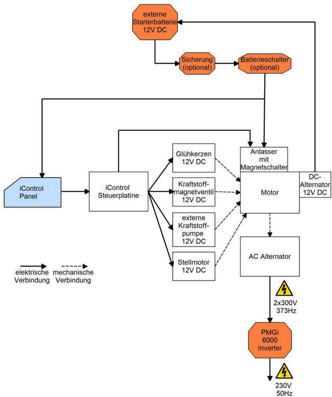
Fig. 7.3.4-1: Elektrisches System
