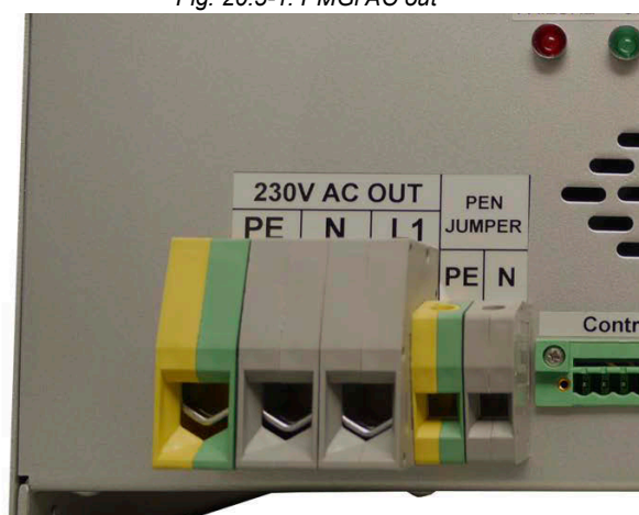
Fig. 20.5-1: PMGi AC out
