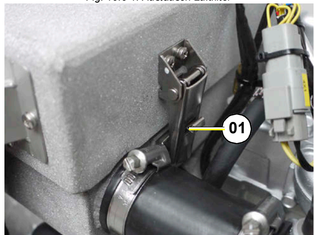
Fig. 10.6-1: Austausch Luftfilter
