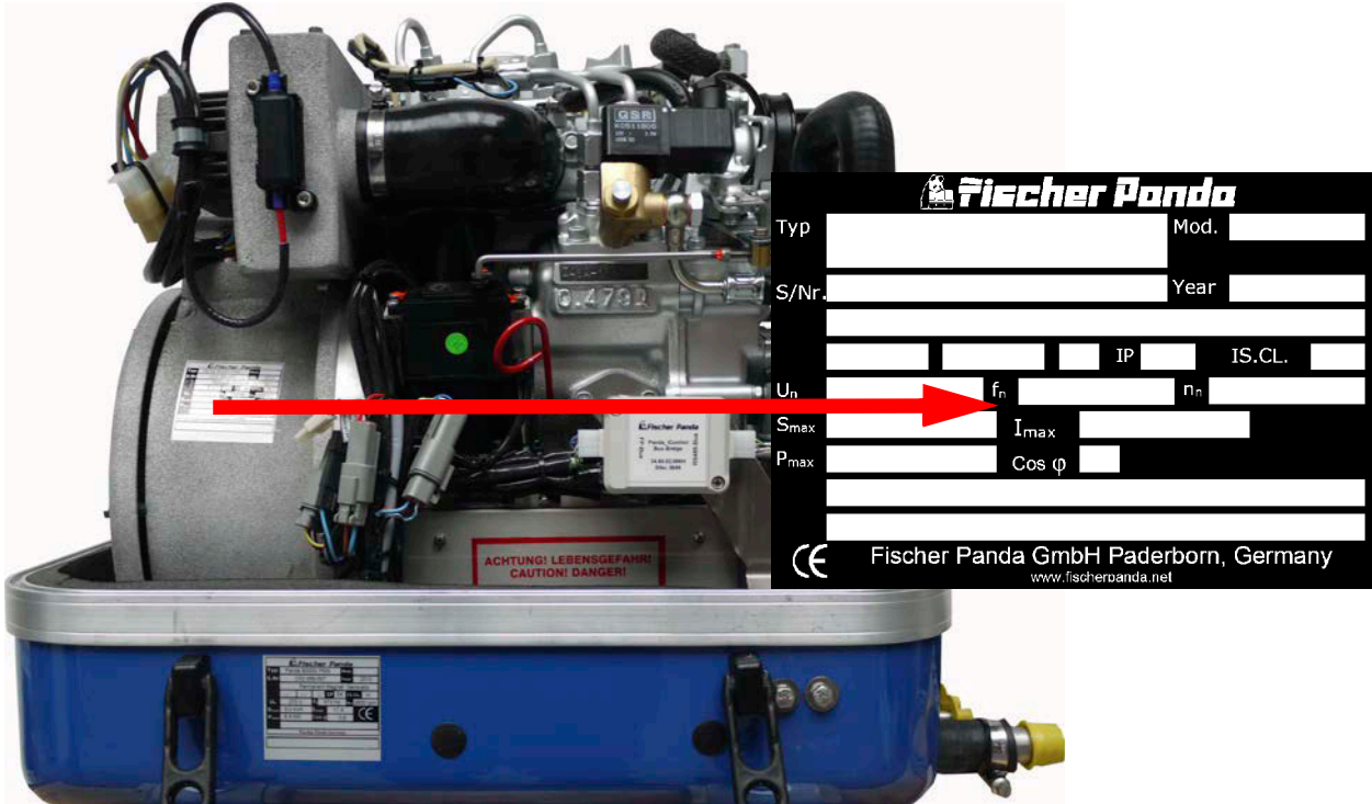
Fig. 7.1-2: Typenschildbeschreibung
