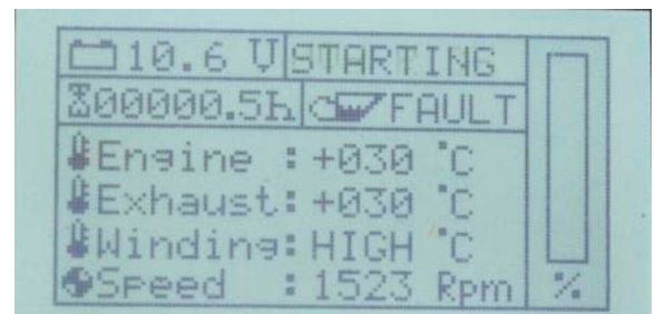
Fig. 18.1.1-2: Warnung „Wicklung“ zu hoch“
