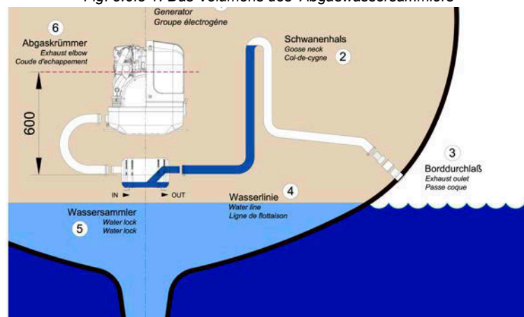
Fig. 8.6.3-1: Das Volumen des Abgaswassersammlers
