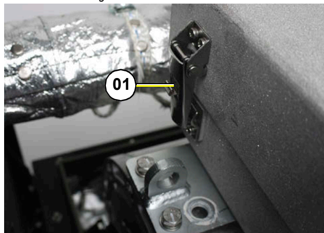
Fig. 10.6-3: Austausch Luftfilter
