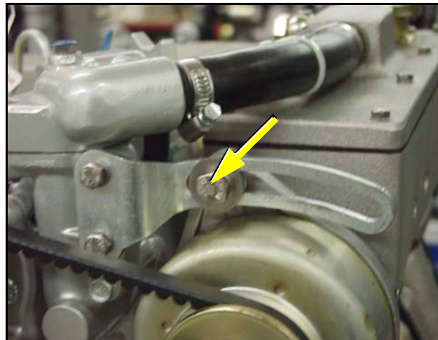
Fig. 10.13-2: Schraube unter der Lichtmaschine
