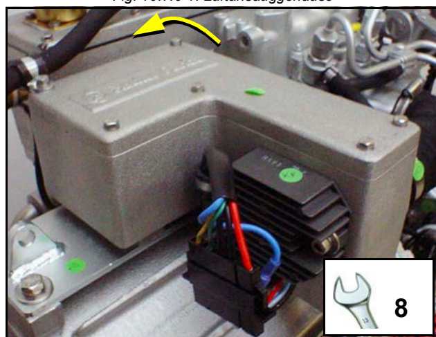
Fig. 10.7.0-1: Luftansauggehäuse
