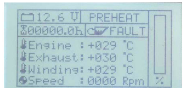
Fig. 15.3.3.2-1: Standard-Displayseite während des Vorglühens
