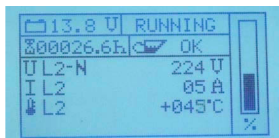
Fig. 15.3.3.4-6: Phasenspannung L2
