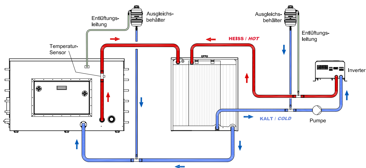
Fig. 20.11.1.3-1: Kühlwasserschema wenn der Radiator auf gleicher höhe oder niedriger als der Generator
