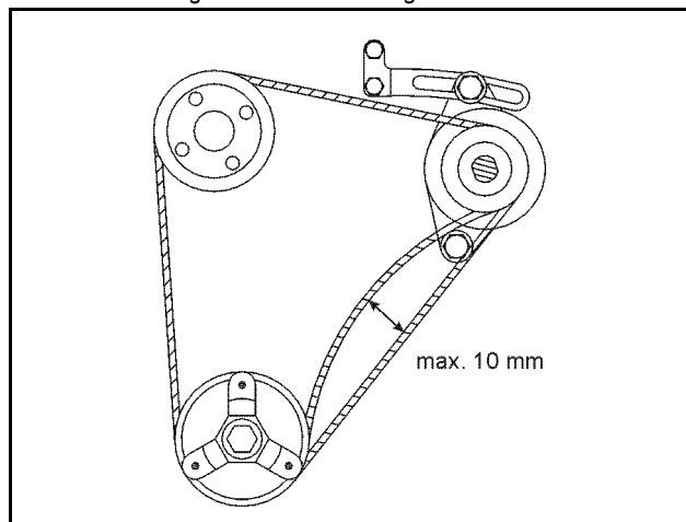
Fig. 10.13-4: Zeichnung Keilriemen
