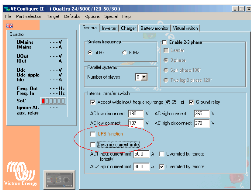
Fig. 20.7.1-1: Einstellungen in der Victron VE configure II Software
