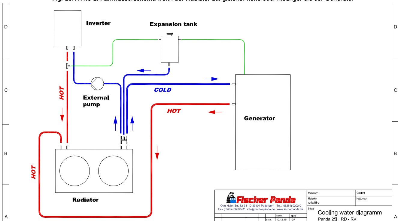
Fig. 20.11.1.3-2: Kühlwasserschema wenn der Radiator auf gleicher Höhe oder niedriger als der Generator
