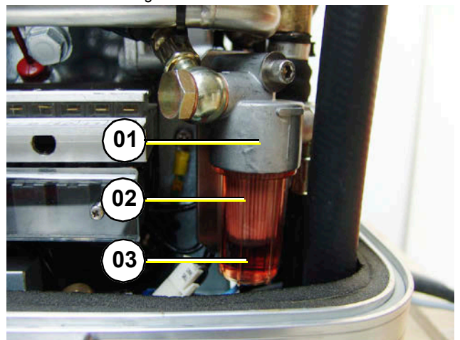
Fig. 10.7.3.1-1: Kraftstofffilter
