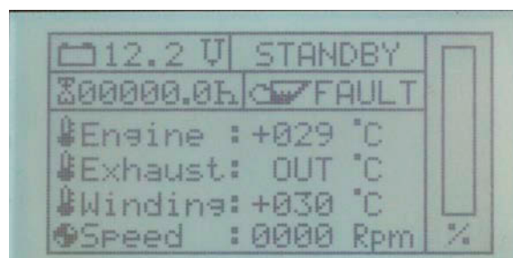
Fig. 18.2.0-1: Fehler „Zylinderkopftemperatur out of range“
