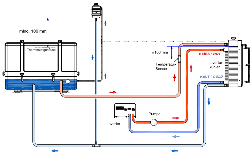
Fig. 20.11.1.2-1: Kühlwasserschema mit dem Radiator höher als der Generator
