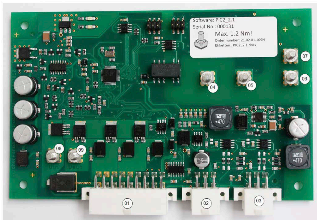
Fig. 16.4-1: Beschaltung des Panda iControl2-Steuergerätes
