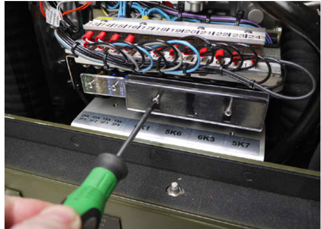
Fig. 10.11-1: Relais
