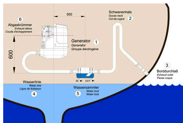
Fig. 8.6.3.2-1: Wassersammler 500 mm neben der Mittellinie des Generators
