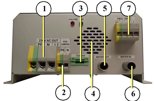
Fig. 13.3-1: Anschlusseite
