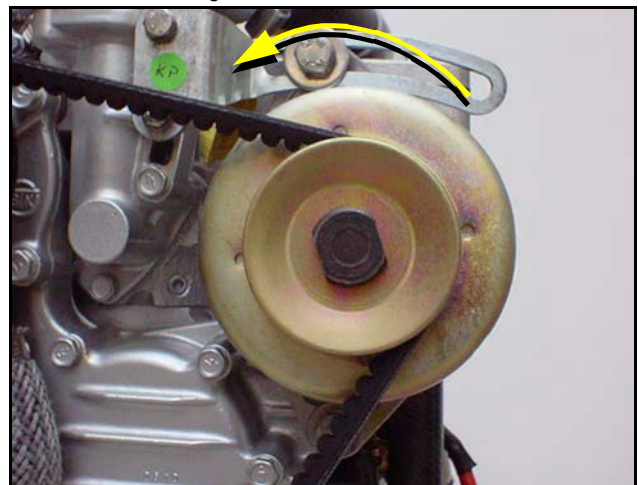
Fig. 10.13-3: Lichtmaschine
