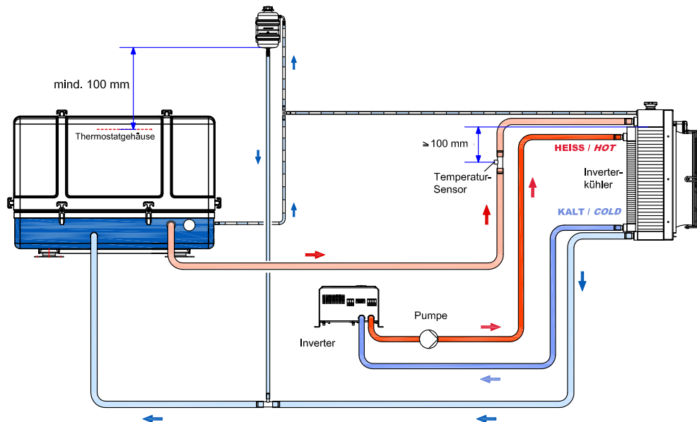
Fig. 13.11.1.2-1: Kühlwasserschema mit dem Radiator höher als der Generator
