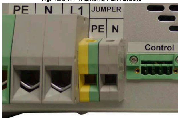
Fig. 13.5.1.4-1: Externe PE/N Brücke
