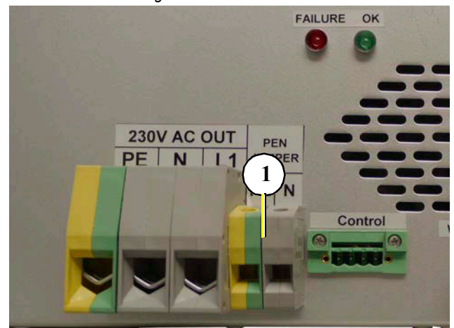
Fig. 13.11-1: PE-N Brücke
