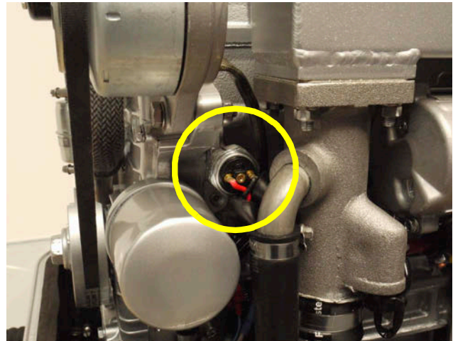
Fig. 7.3.6-4: Öldruckschalter
