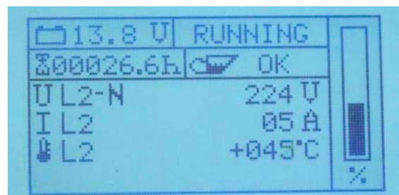
Fig. 15.3.3.4-6: Phasenspannung L2
