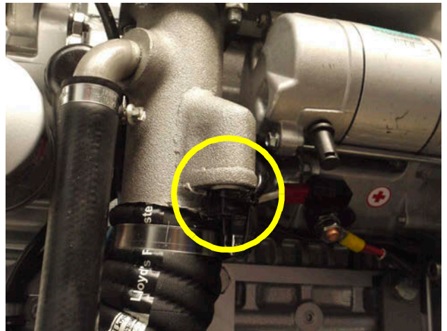
Fig. 7.3.6-2: Thermosensor am Abgaskrümmmer
