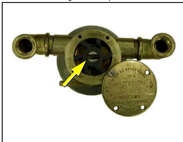
Fig. 10.4.3-4: Impeller
