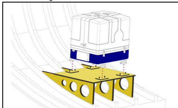
Fig. 8.2.3-1: Generator-Fundament
