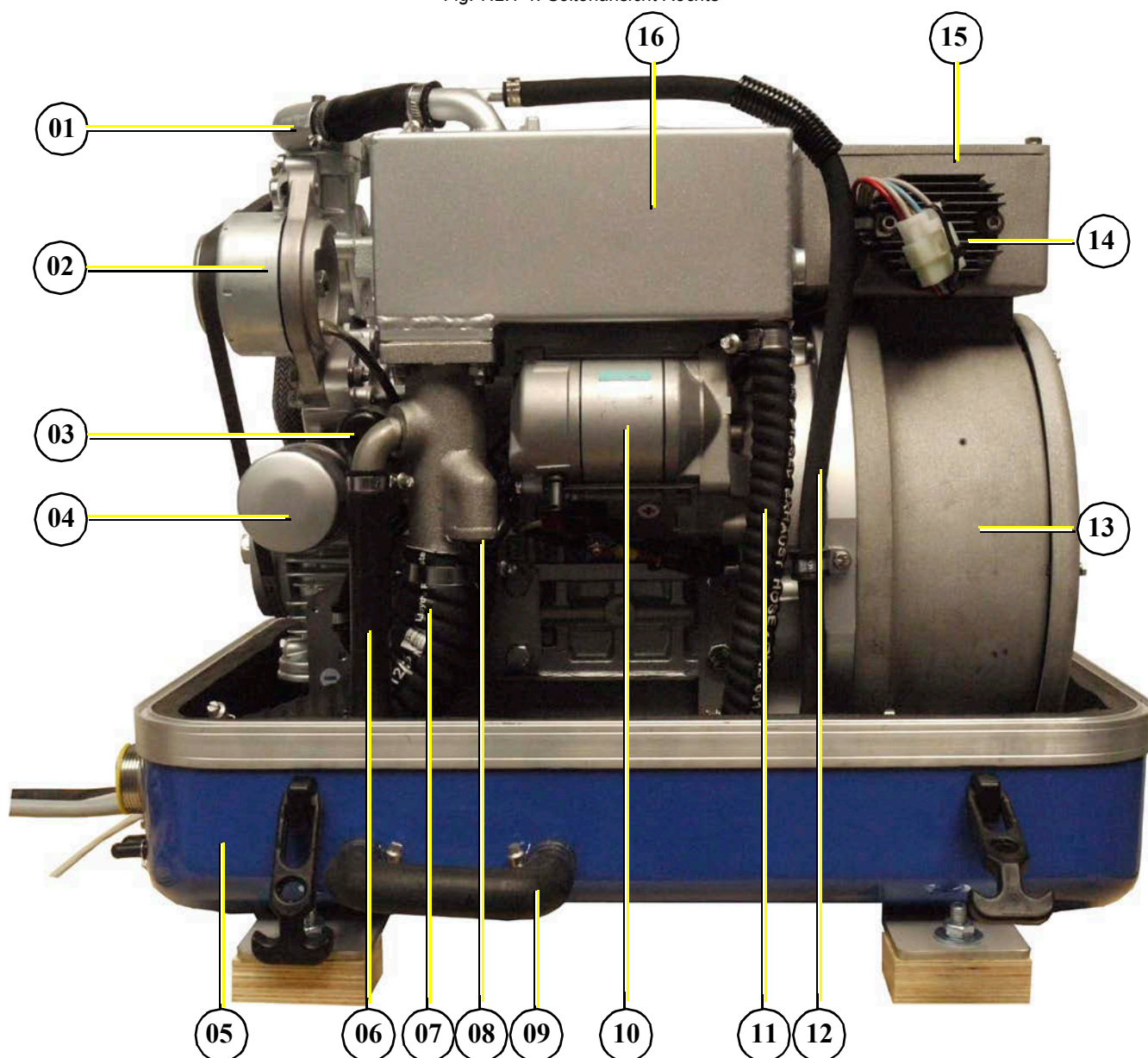
Fig. 7.2.1-1: Seitenansicht Rechts
