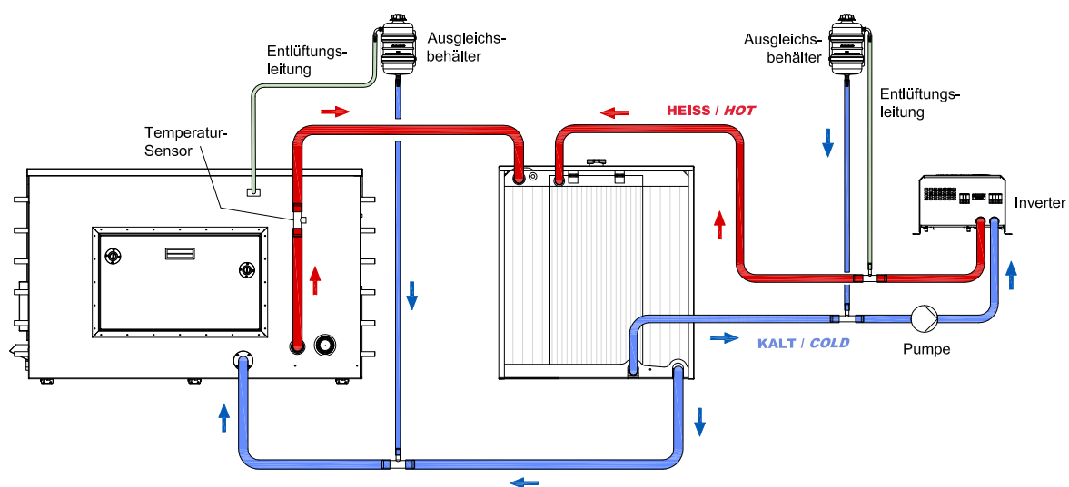
Fig. 13.11.1.3-1: Kühlwasserschema wenn der Radiator auf gleicher höhe oder niedriger als der Generator
