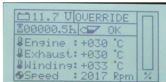
Fig. 15.3.3.3-1: Standard-Displayseite während des Override-Modus
