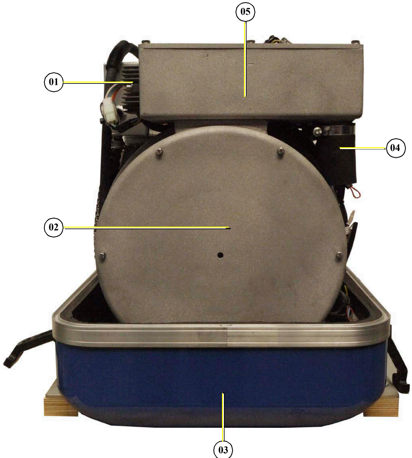
Fig. 7.2.4-1: Rückseite
