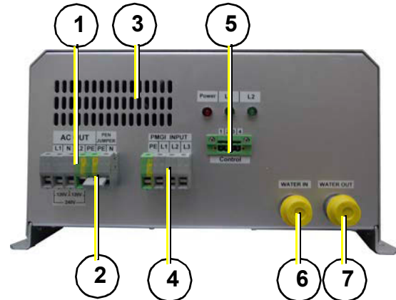
Fig. 13.5-1: Anschlusseite
