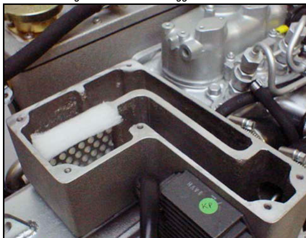
Fig. 10.7.0-2: Luftansauggehäuse offen
