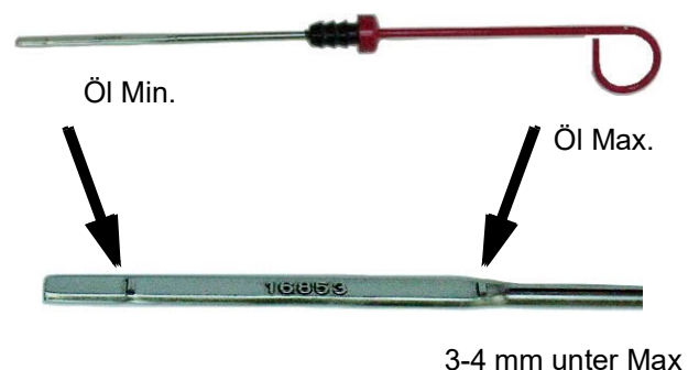
Fig. 10.8.1-1: Ölpeilstab - Beispiel
