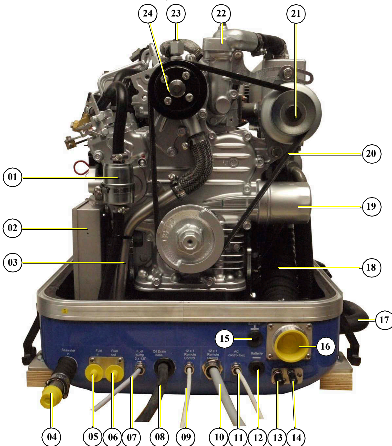
Fig. 7.2.3-1: Vorderseite
