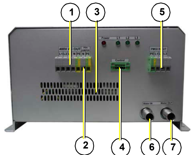
Fig. 13.4-1: Anschlusseite
