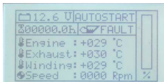
Fig. 15.4.6-7: Standard-Displayseite im Autostart-Modus
