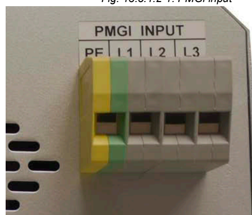
Fig. 13.5.1.2-1: PMGi input
