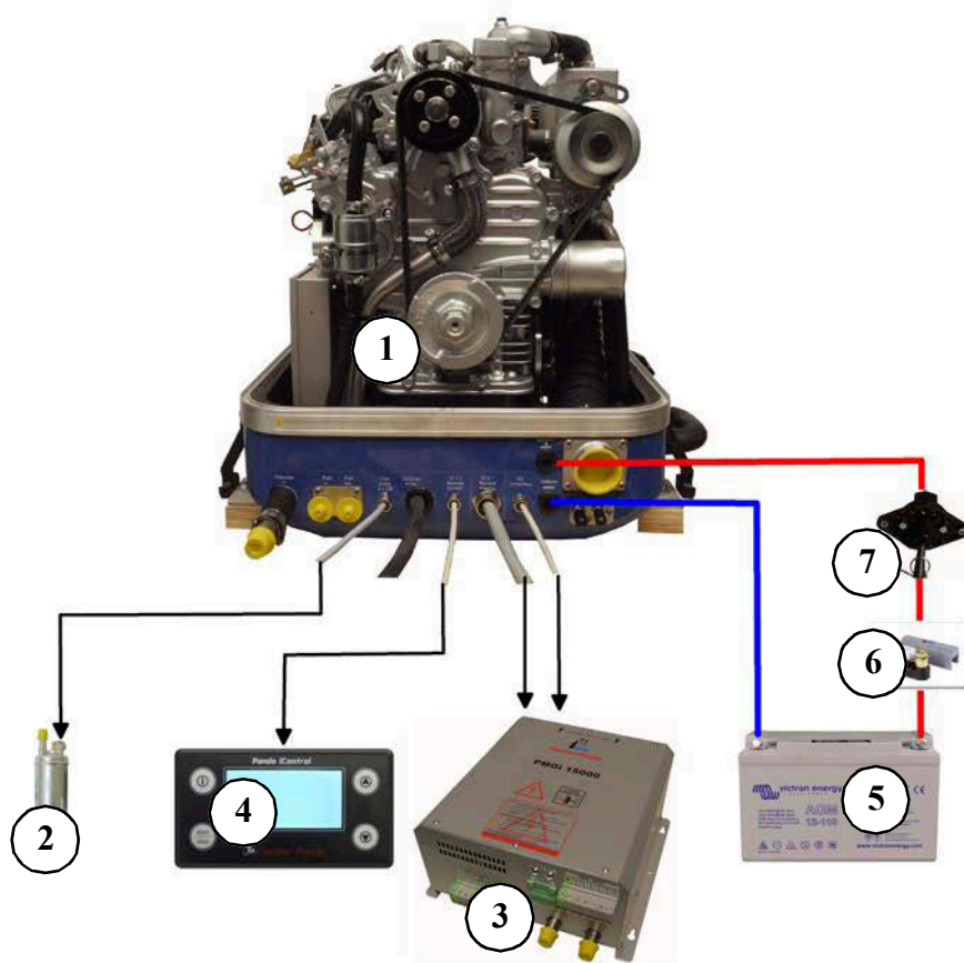
Fig. 8.12.0-1: Installationsschema Beispiel
