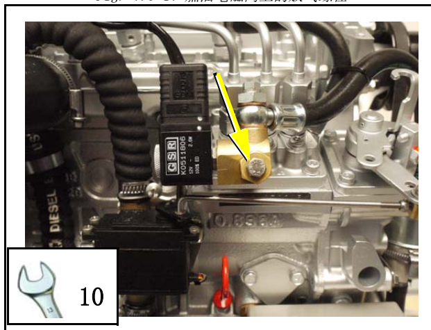
Fig. 7.9-1: 燃油电磁阀上的放气螺栓
