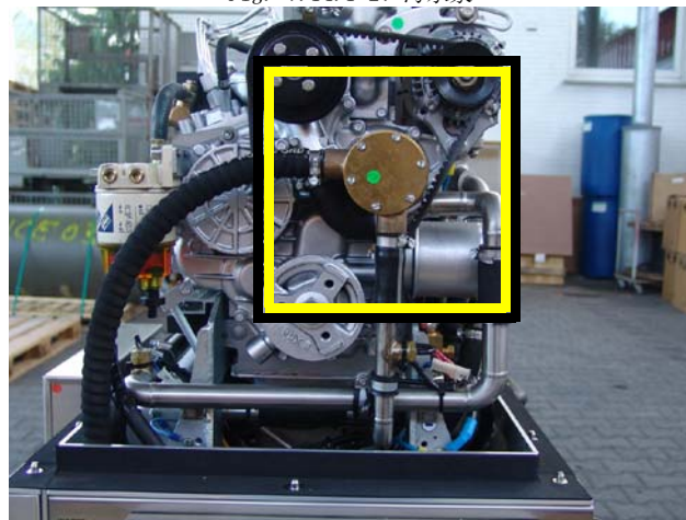
Fig. 7.14.1-3: 海水泵盖
