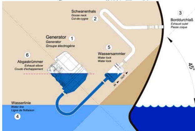
Fig. 5.7.3.2-2: 倾斜位置 45 度
