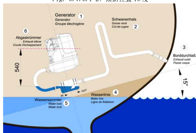
Fig. 5.7.3.1-2: 倾斜位置 15 度
