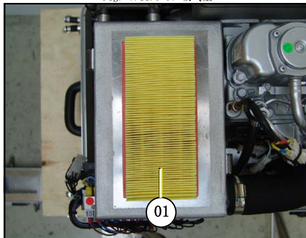
Fig. 7.11.3-3: 吸气室
