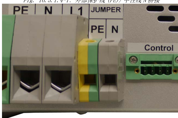
Fig. 16.5.1.4-1: 外部保护线 (PE)/ 中性线 N 桥接
