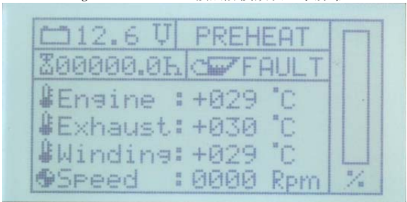
Fig. 11.3.3.2-1: 预热阶段默认显示屏幕
