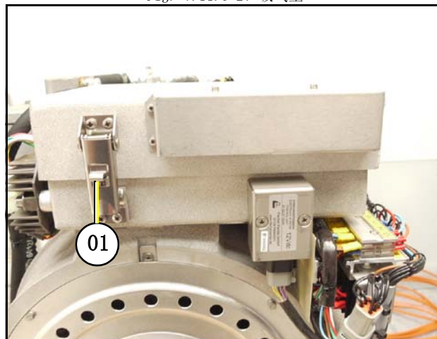
Fig. 7.11.3-2: 吸气室
