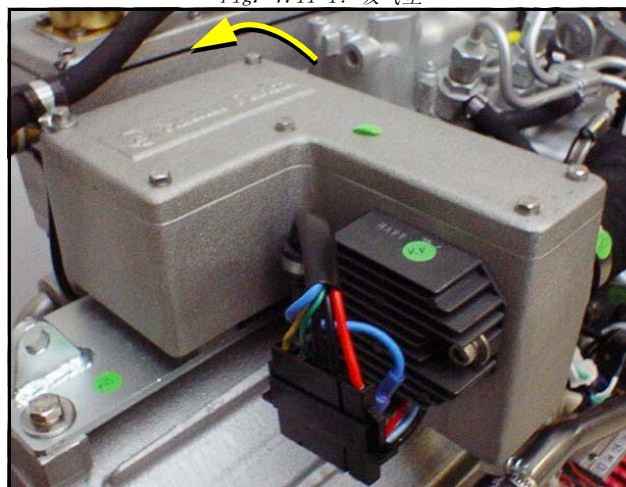
Fig. 7.11-1: 吸气室
