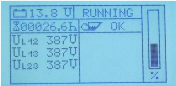
Fig. 11.3.3.4-4: 转换器屏幕 线电压
