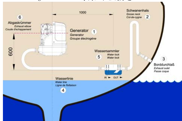
Fig. 5.7.3.2-3: 水封, 中心线旁边 1000 mm
