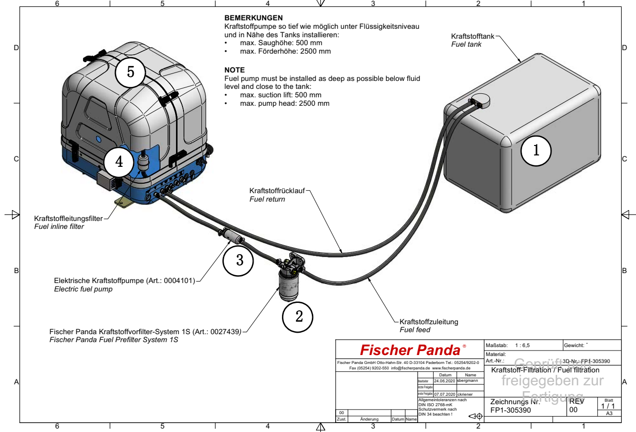
Fig. 5.10.1-2: 燃油系统 - 示意图
