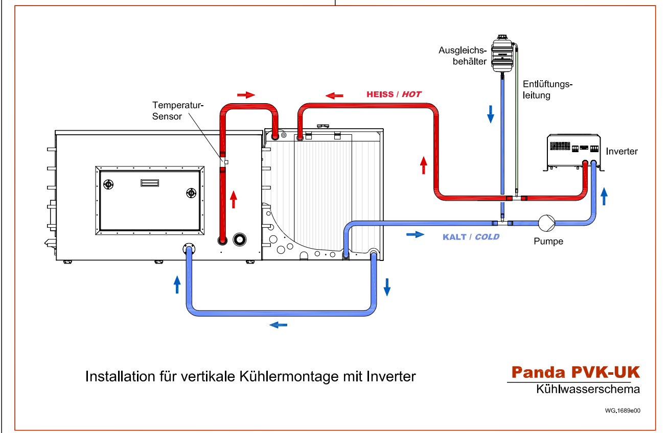
Fig. 16.11.1.4-1: i 系列发电机组 (PVK-UK) 冷却水示意图
