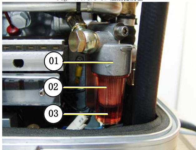
Fig. 7.9.1.1-2: 燃油滤清器
