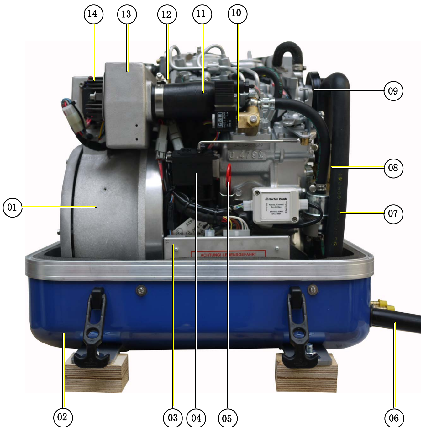
Fig. 4.1.2-1: 左侧视图
