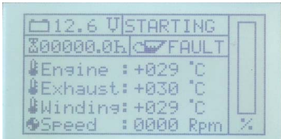
Fig. 11.3.3.2-2: 启动阶段默认显示屏幕
