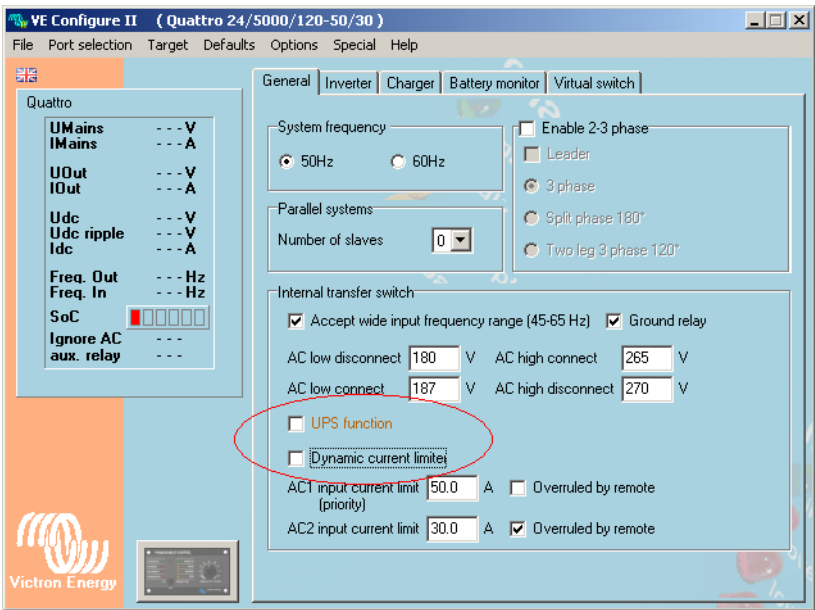
Fig. 16.7.1-1: 维克特龙 (Victron) VE 配置 II 软件中的设置
