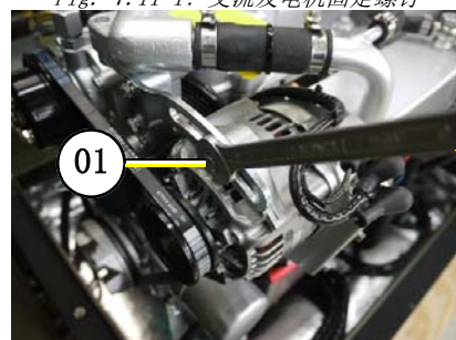
Fig. 7.11-2: 交流发电机固定螺钉
