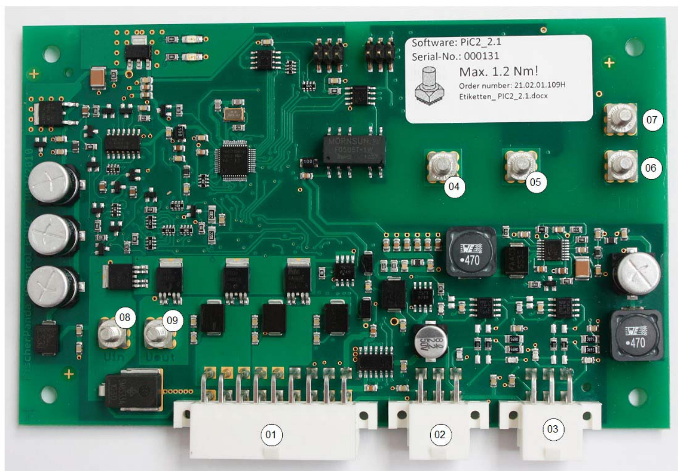
Fig. 12.4-1: Panda iControl2 控制器接线
