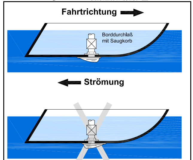
Fig. 5.4.2-1: 贯穿船体配件的位置
