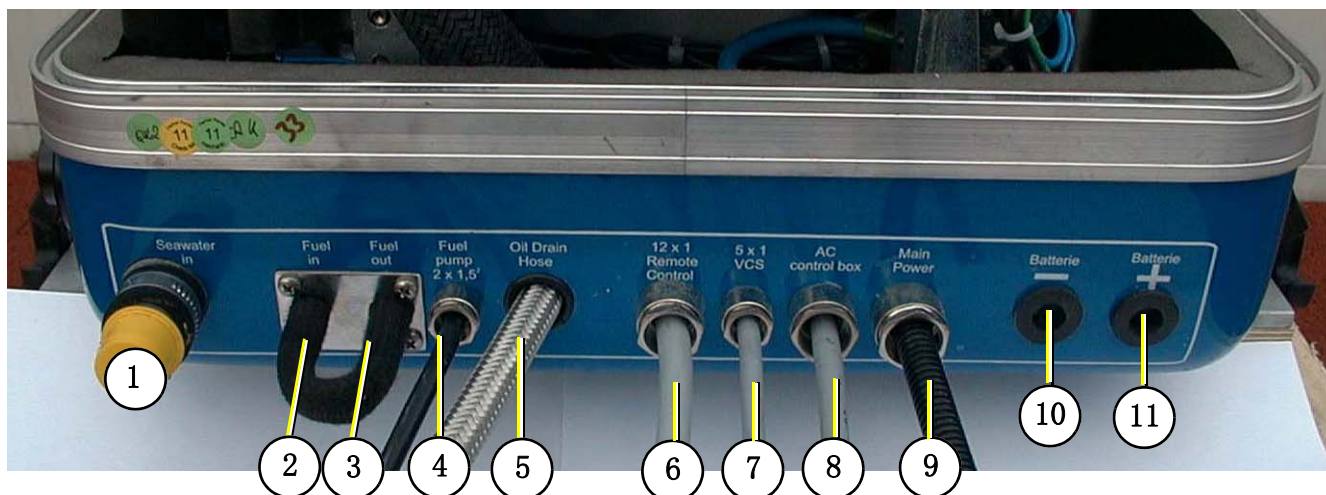
Fig. 5.3-1: 发电机连接 - 示例
