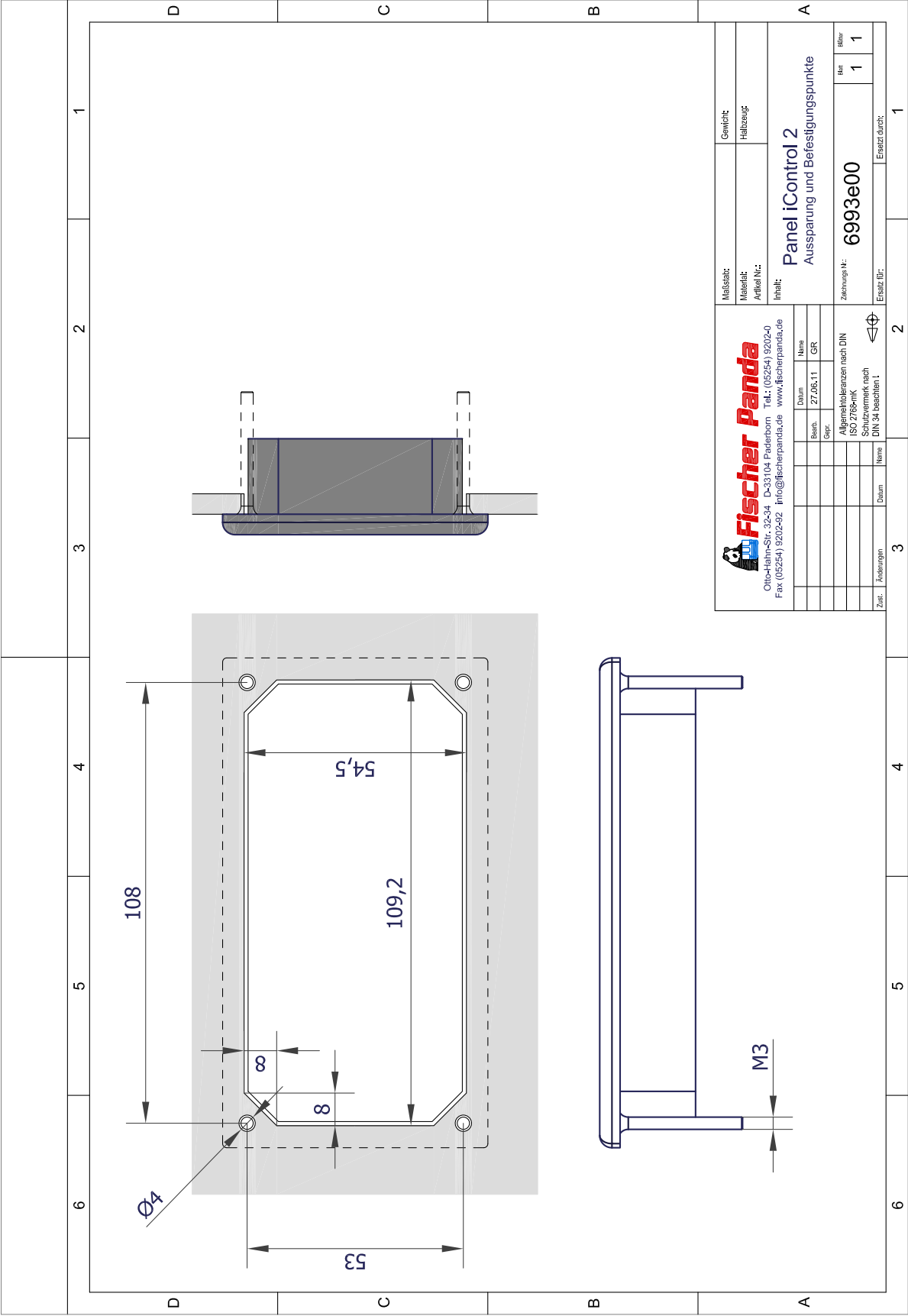
Fig. 12.3-1: Panda iControl2 控制面板外壳
