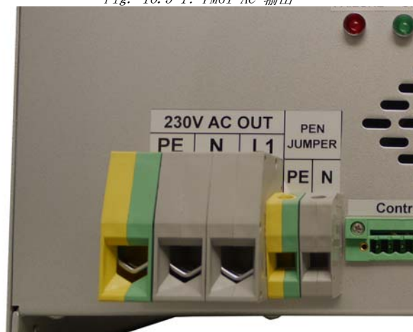
Fig. 16.5-1: PMGi AC 输出
