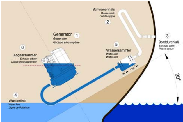
Fig. 5.7.3.2-4: 倾斜位置 30 度
