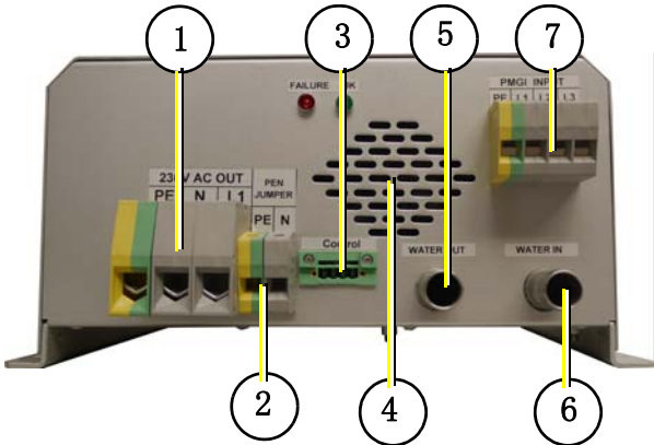
Fig. 16.3-1: 连接侧
