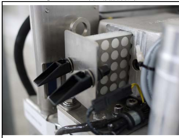
Fig. 7.11.2-3: 带拉出支架的吸气室
