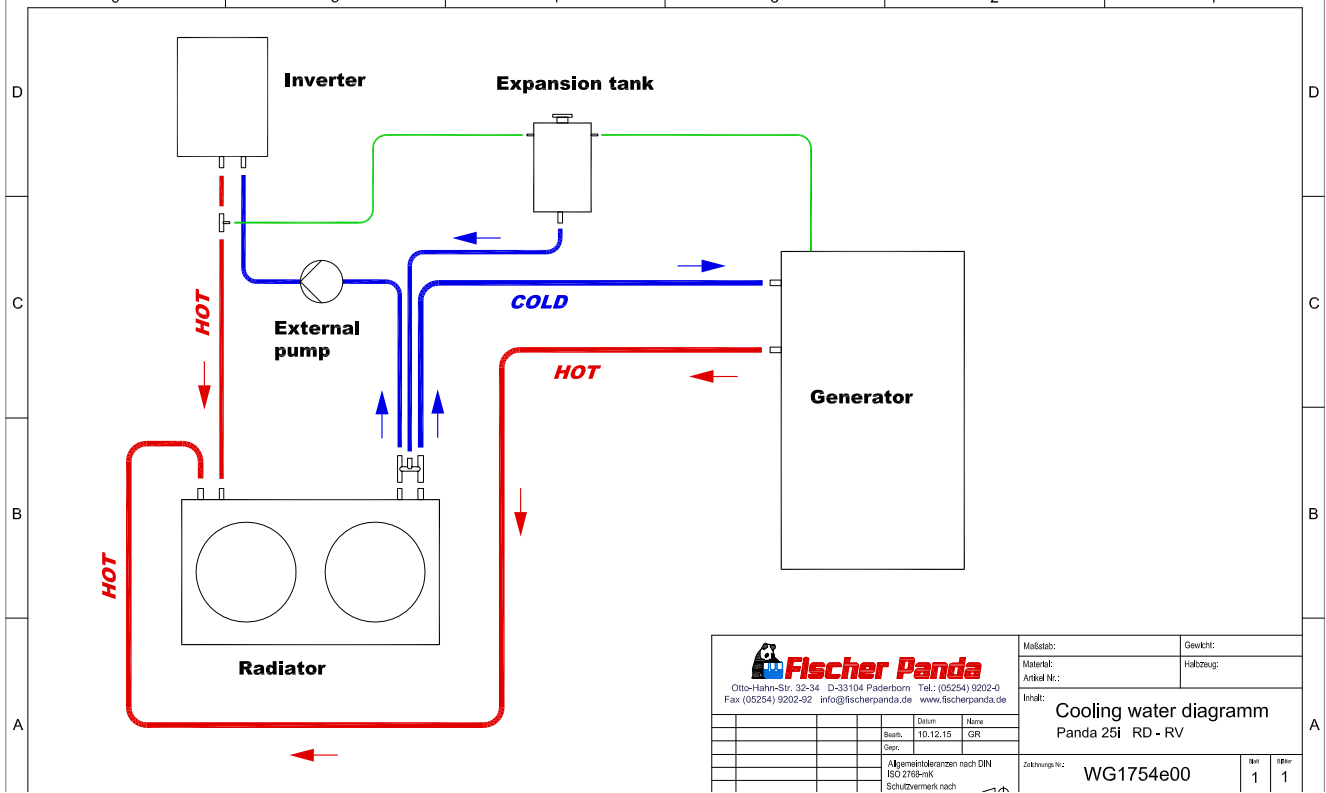
Fig. 16.11.1-2: 如果散热器与发电机 / 逆变器处于相同高度或更低水冷却示意图
