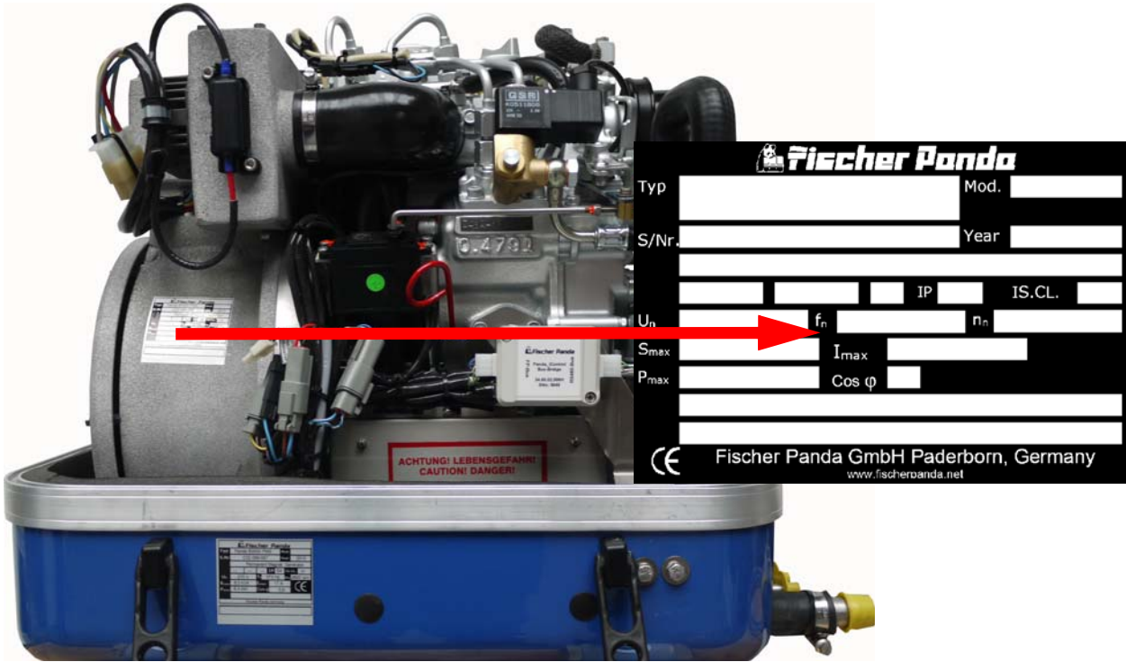
Fig. 4.1-2: 铭牌描述
