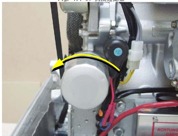
Fig. 7.7-3: 机油过滤器
