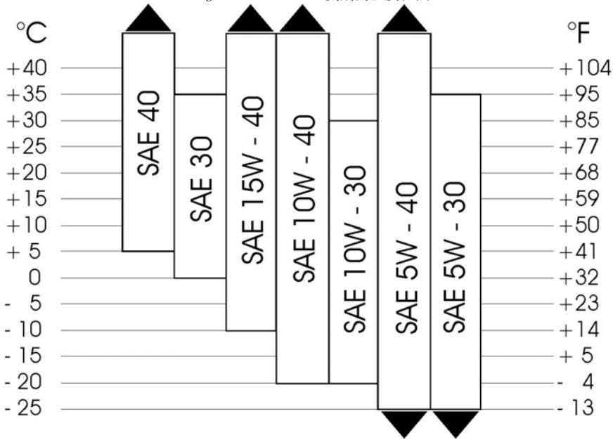
Fig. 9.5.1-2: SAE 类别的温度范围
