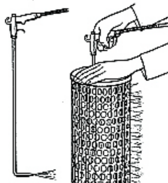
Fig. 7.12-8: 清洁空气过滤器
