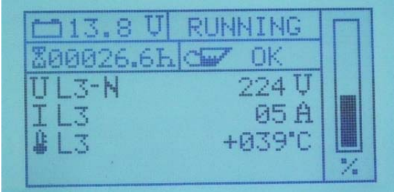
Fig. 11.3.3.4-7: 相电压 L3
