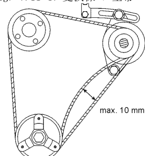
Fig. 7.11-4: 更换保 V 型带
