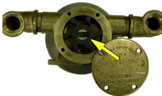
Fig. 7.14.1-4: 叶轮泵
