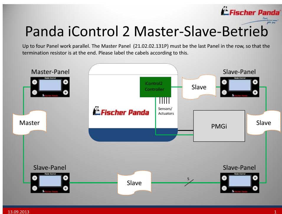
Fig. 12.5-1: 主从面板配置
