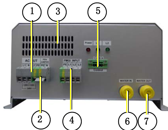
Fig. 16.5-1: 连接侧
