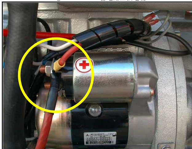
Fig. 5.11.2-1: 蓄电池正极电缆
