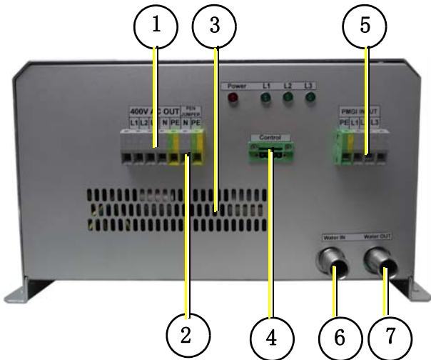
Fig. 16.4-1: 连接侧
