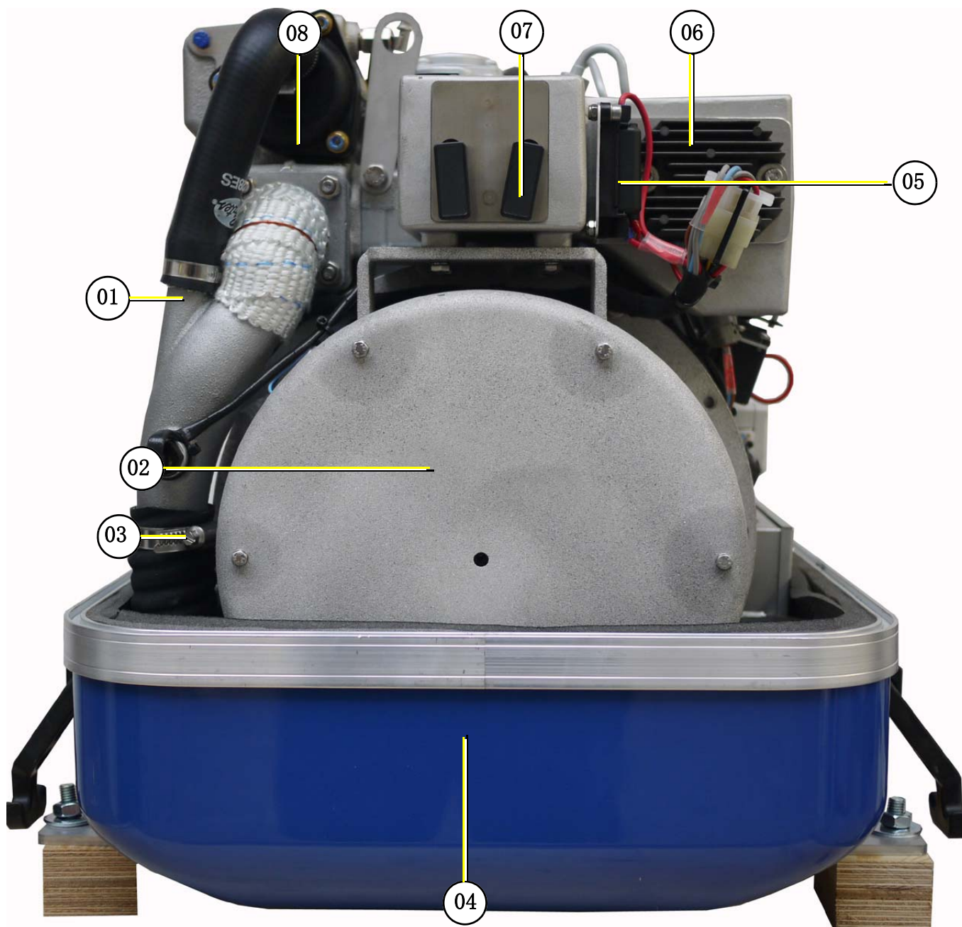
Fig. 4.1.4-1: 后视图
