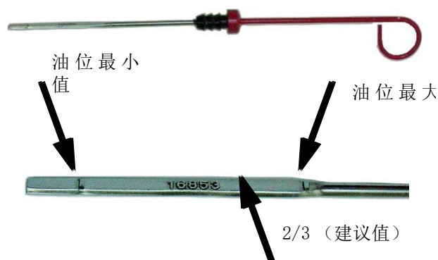
Fig. 7.6-1: 机油尺 - 样品
