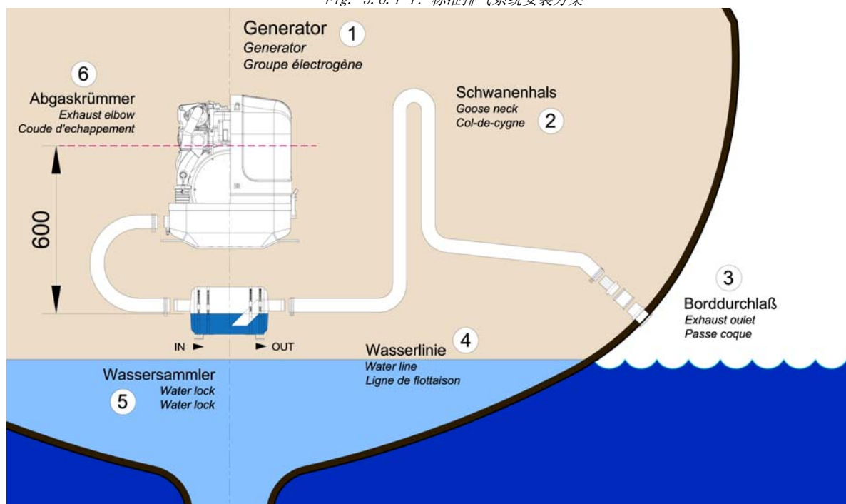
Fig. 5.6.1-1: 标准排气系统安装方案
