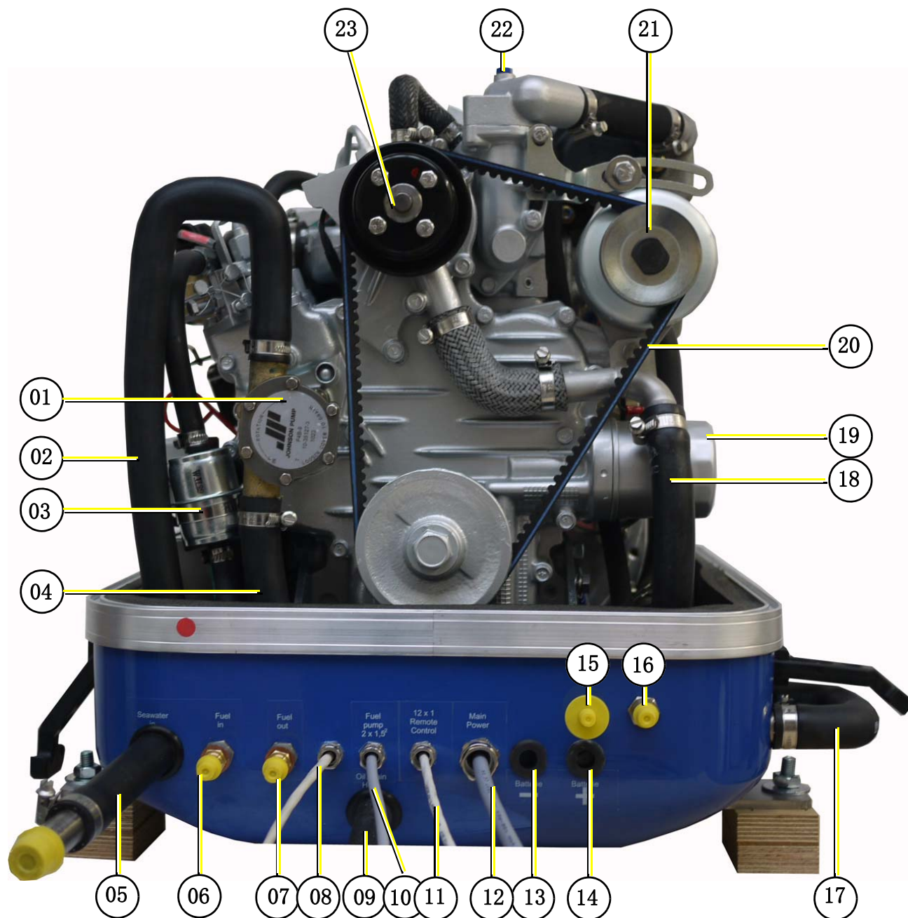
Fig. 4.1.3-1: 正视图
