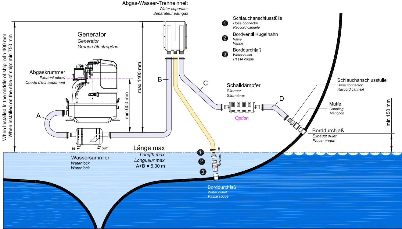
Fig. 5.8-1: 排气 / 水分离器安装方案
