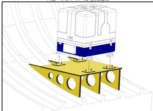
Fig. 5.2.3-1: 发电机底座
