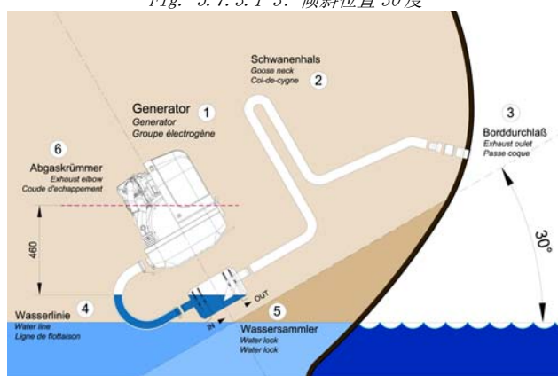
Fig. 5.7.3.1-3: 倾斜位置 30 度
