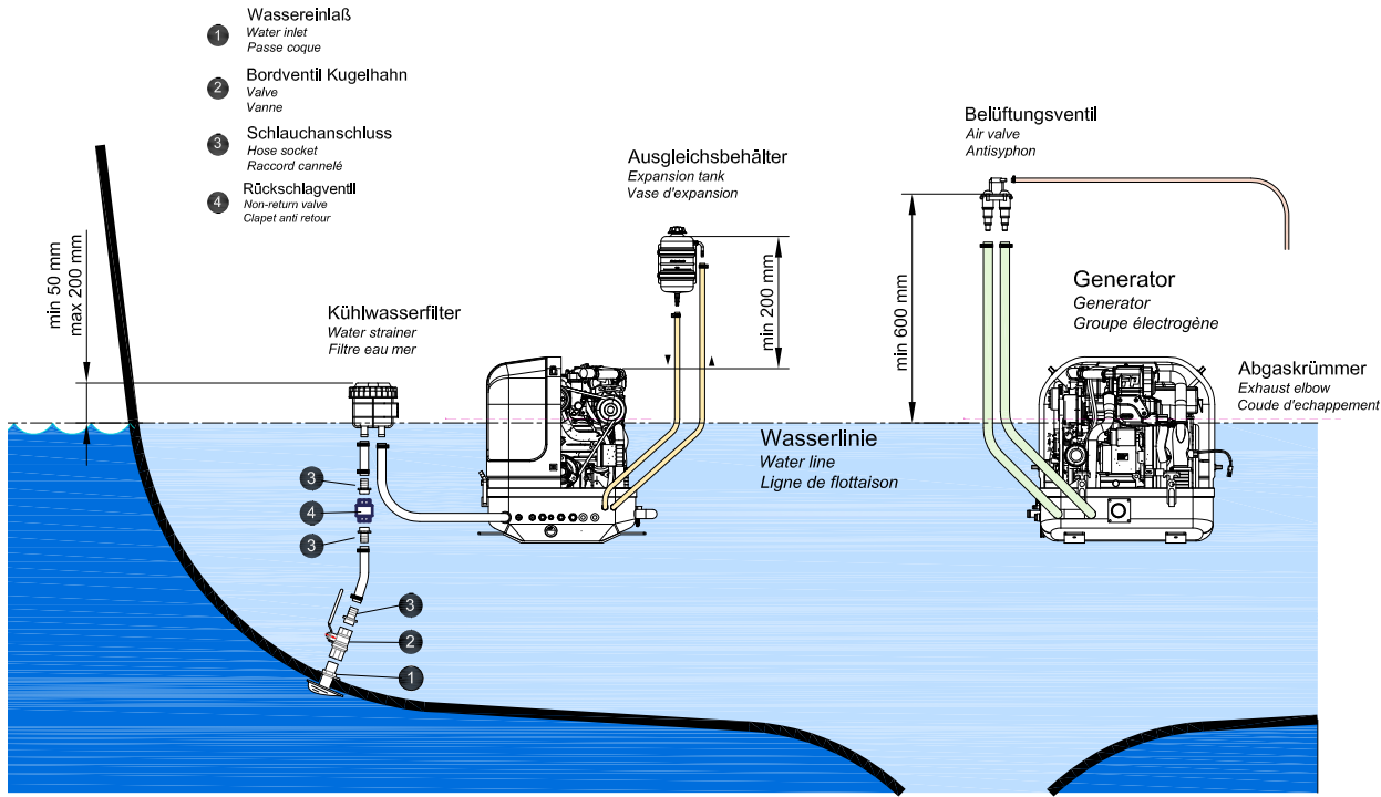
Fig. 5.4.5.1-1: 海水安装方案
