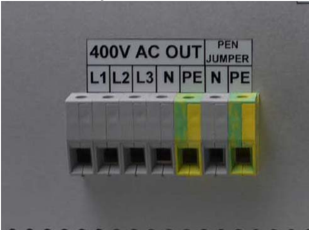
Fig. 16.5-3: PMGi AC 输出
