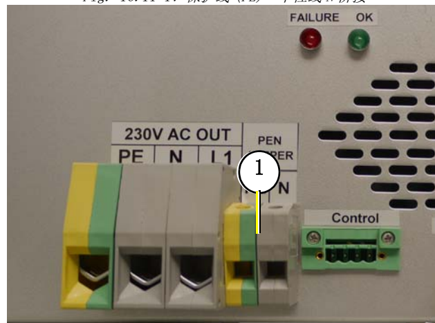
Fig. 16.11-1: 保护线 (PE)– 中性线 N 桥接
