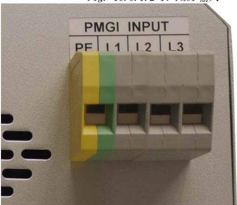
Fig. 16.5.1.2-1: PMGi 输入
