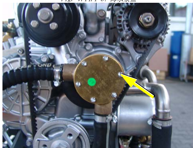
Fig. 7.14.1-3: 海水泵盖
