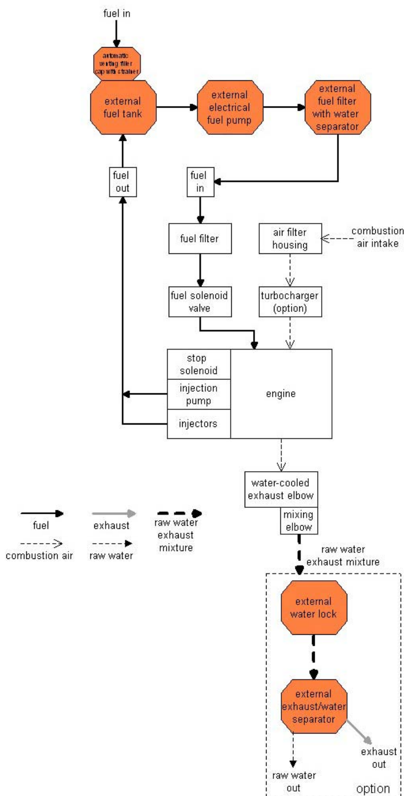
Fig. 4.2.3-1: 燃油、进气和排气系统
