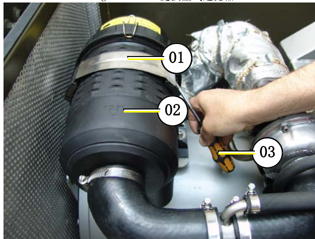
Fig. 7.12-2: 更换空气过滤器
