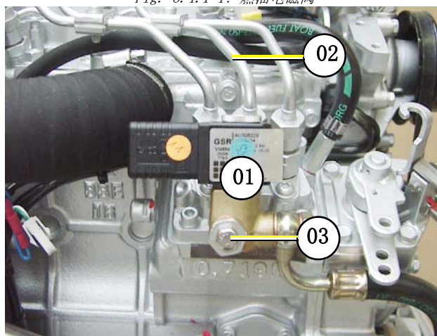
Fig. 8.4.1-1: 燃油电磁阀
