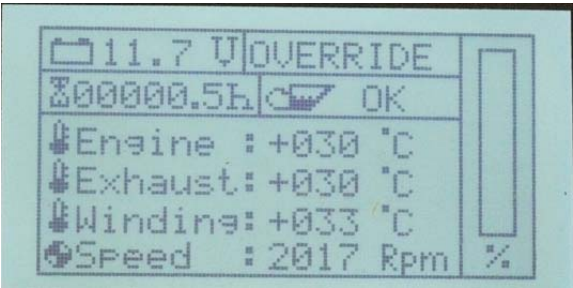
Fig. 11.3.3-1: 重写（覆盖）模式默认显示屏幕
