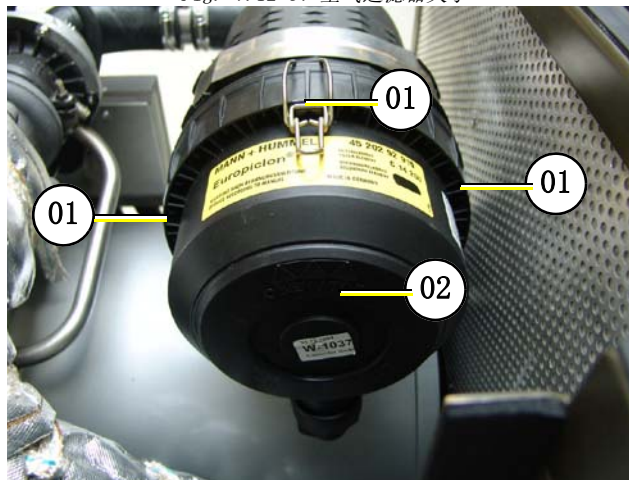
Fig. 7.12-3: 空气过滤器夹子
