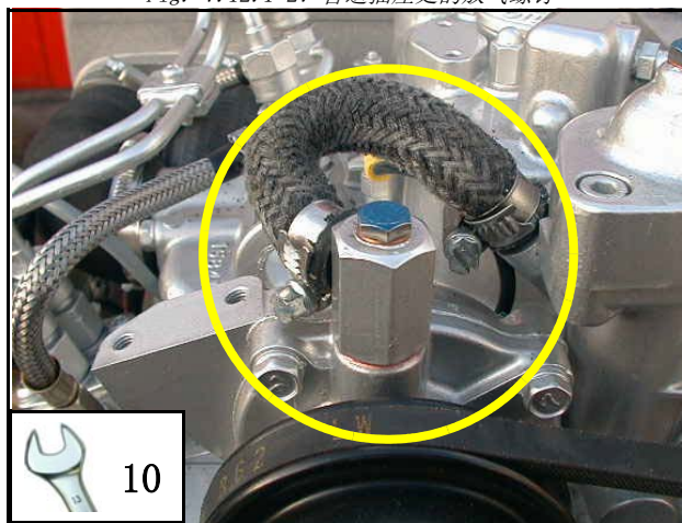
Fig. 7.12.1-2: 管道插座处的放气螺钉
