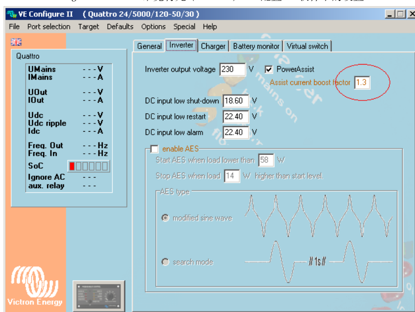
Fig. 16.7.2-1: 维克特龙 (Victron) VE 配置 II 软件中的设置
