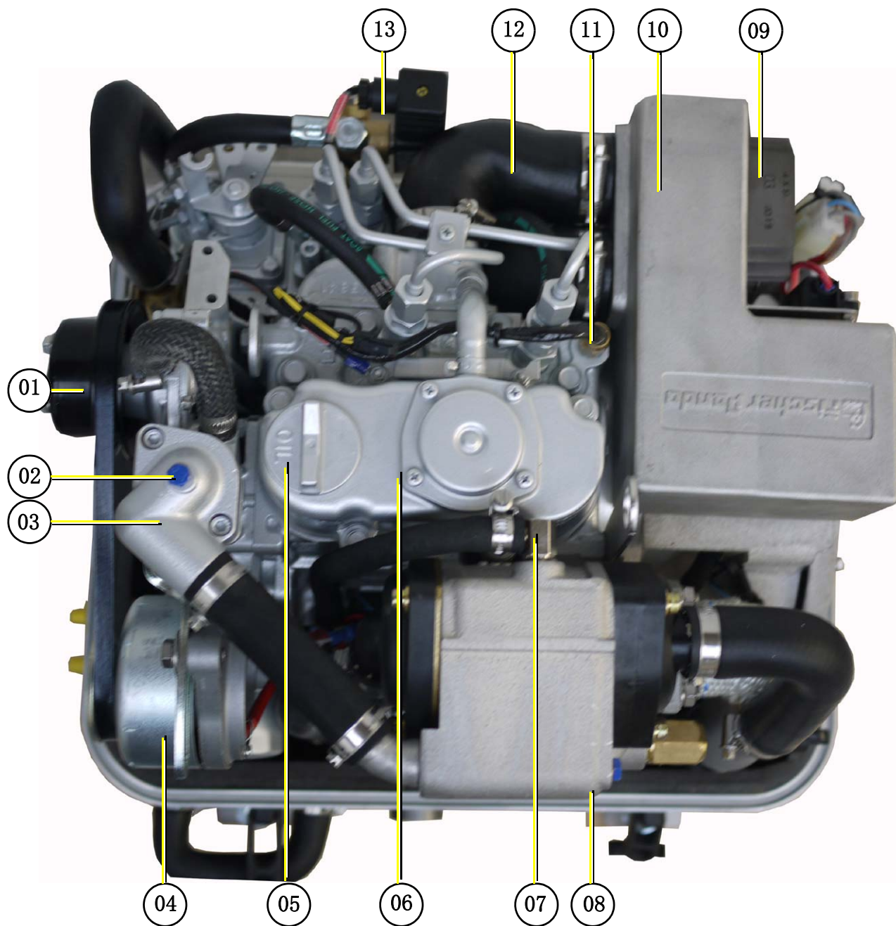
Fig. 4.1.5-1: 顶视图
