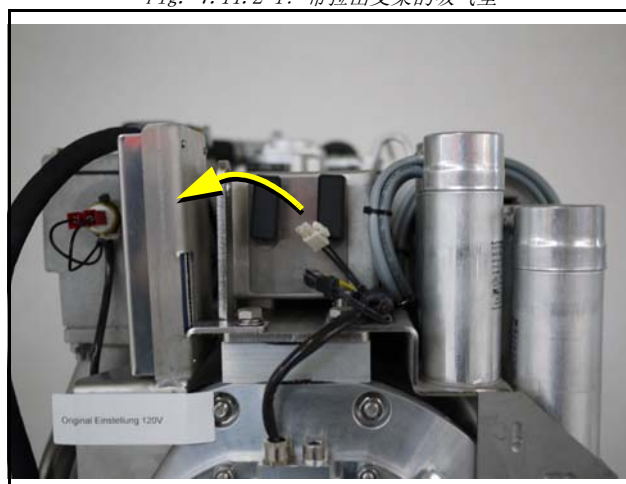
Fig. 7.11.2-1: 带拉出支架的吸气室
